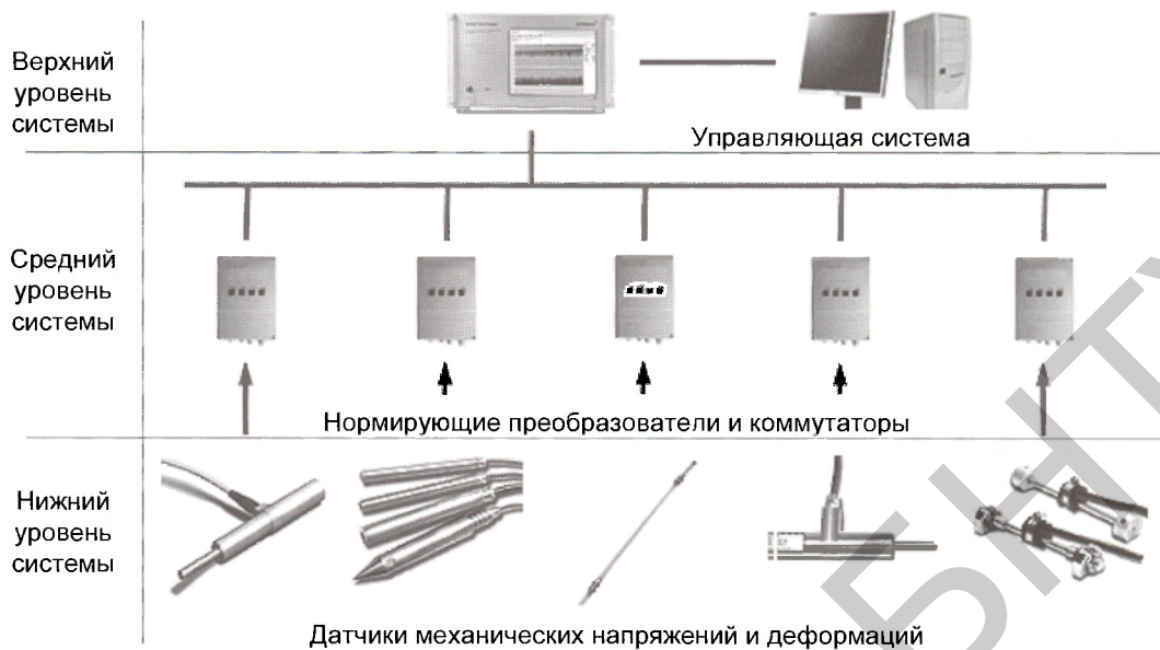
Рис. 2. Типовая структура системы строительного мониторинга
