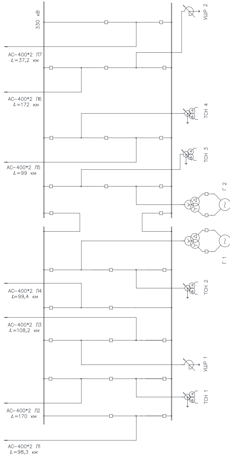
Рис. 1. Главная схема электрических соединений атомной электростанции: Л – воздушная линия электропередачи; ТСН – трансформатор собственных нужд; Г – генератор; УШР – управляемый шунтирующий реактор Fig. 1. The main wiring circuit of a nuclear power plant: Л – overhead transmission line; ТСН – auxiliary transformer; Г – generator; УШР – controlled shunt reactor
