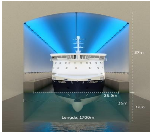
Рисунок 3 – Размеры тоннеля
