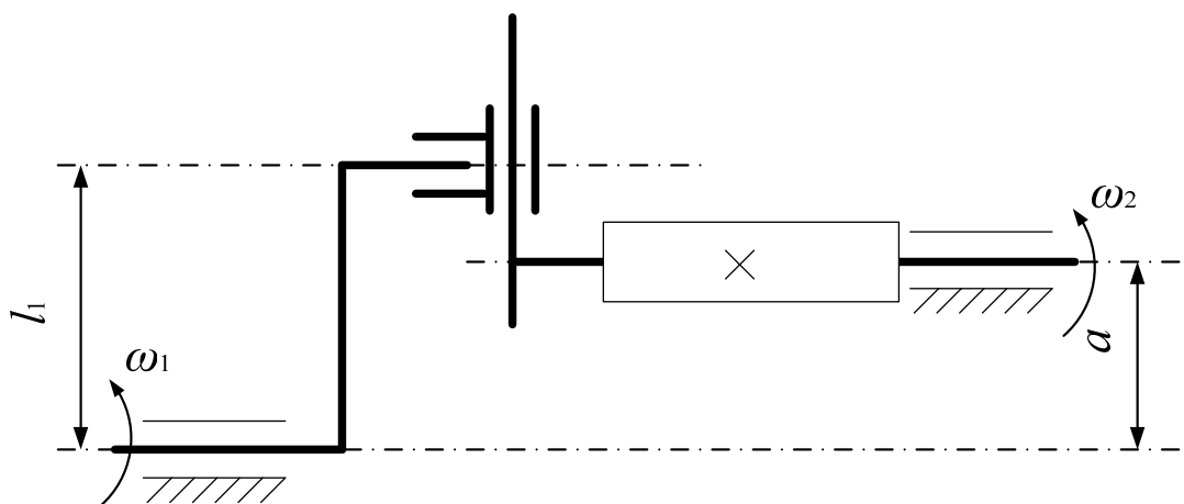
Рис. 3. Схема кулисного механизма привода вращения упрочняемой детали
