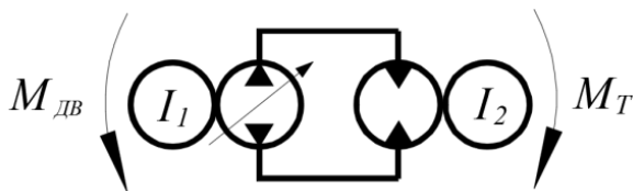
Рисунок 2 – Расчетная схема трансмиссии при торможении через гидропередачу
