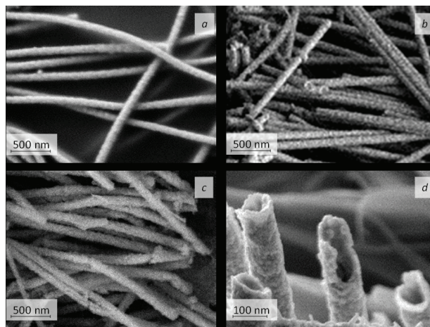
Рисунок 1 – СЭМ-изображения массива ферромагнитных нанотрубок после растворения ПЭТФ-шаблона: a – Fe; b – Co; c – Ni; d – сломы отдельных Ni нанотрубок
