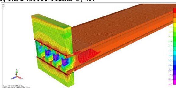
Рисунок 9 – Распределение нормальных напряжений \sigma_y при P = 300 кН
