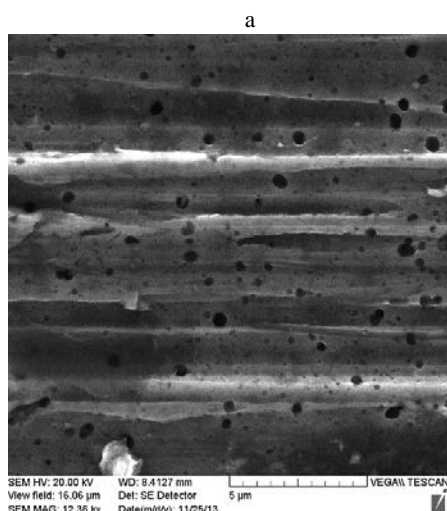
Рис. 12. Поверхность зоны 5 образца, полученного при добавочной индуктивности 3L, напряжении 240 В, концентрации электролита 8 % и температуре 40 °С: а – морфология поверхности; б – микропрофиль поверхности Fig. 12. Zone-5 surface of sample obtained with 3L additional inductance, 240 V voltage, 8 % electrolyte concentration and 40 °C temperature: a – surface morphology; b – surface microprofile
