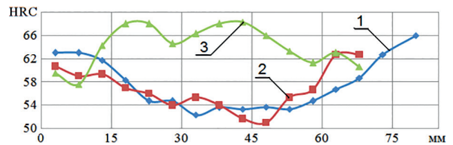
Рис. 6. Характер изменения твердости по толщине отбойных плит: 1 – плита УПМ-1,25.001; 2 – УПМ-1,0.001; 3 – УПМ-1,0.001 после ТО
