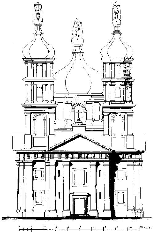
Рис. 3. Главный фасад Успенской церкви в Ушачах
