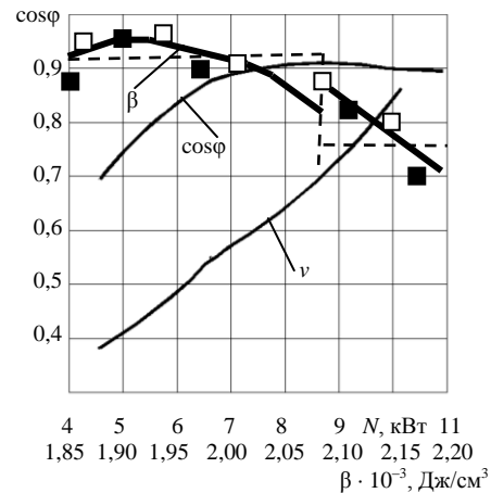
Рис. 2. Зависимость скорости резания от мощности электродвигателя привода главного движения и \cos\varphi , удельной энергоёмкости \beta и \cos\varphi (□ – для образцов D_{\text{заг}} = 32 мм, ■ – для образцов D_{\text{заг}} = 36 мм)
