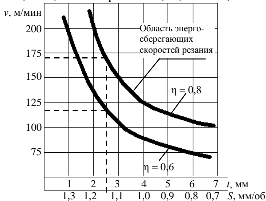
Рис. 1. Зависимость скорости резания от КПД электродвигателя привода главного движения при различных режимах обработки
