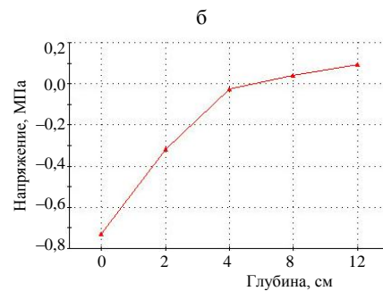
Рис. 5. Результаты моделирования для асфальтобетонных слоев покрытия: а – поле напряжений от действия транспортной нагрузки (жирной линией отмечены границы слоев, сверху вниз – плотный асфальтобетон, пористый асфальтобетон, щебень); б – распределение температурных напряжений с глубиной при действии транспортной нагрузки
