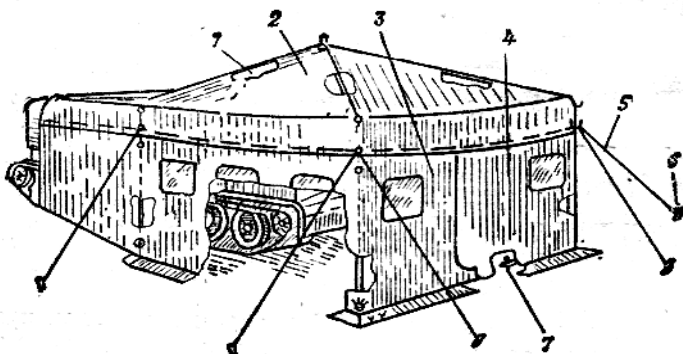
Рис. 2.3 Общий вид палатки: 1 – каркас; 2 – верхний намет; 3 – левый намет; 4 – правый намет; 5 – растяжка; 6 – кол; 7 – приколыш
