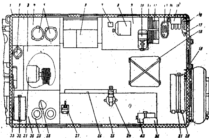
Рис. 2.6. Размещение оборудования и имущества в кузове ремонтно-зарядной аккумуляторной станции СРЗ-А-М1:
