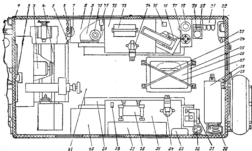
Рис. 2.4. Размещение оборудования и имущества в кузове мастерской МРМ-М1:
