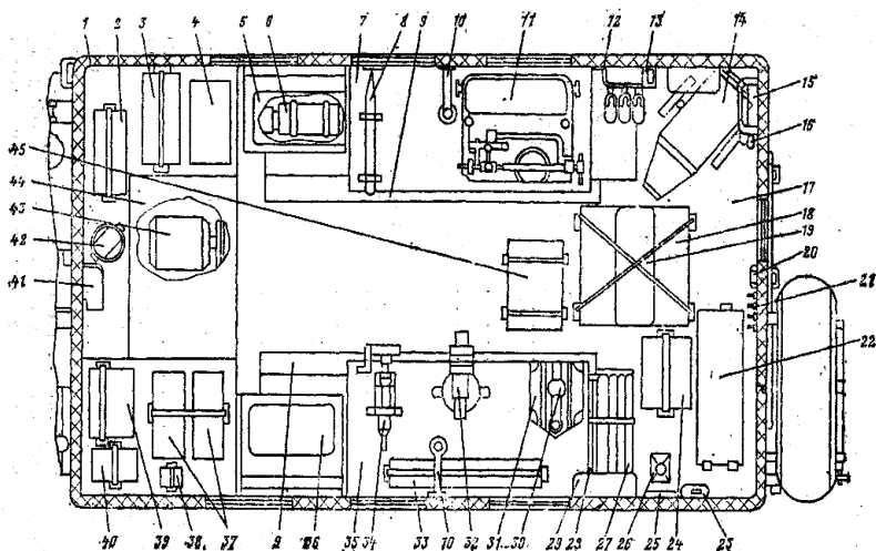
Рис. 2.2 Размещение оборудования и имущества в кузове мастерской MPC-AT-M1:
