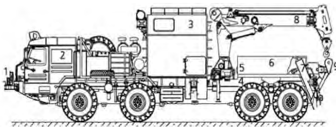
Рис. 3.13 Машина ремонтно-эвакуационная колесная средняя РЭМ-КС:
