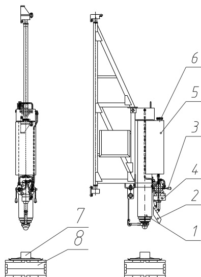
Рис. 4.5. Гидроопора
