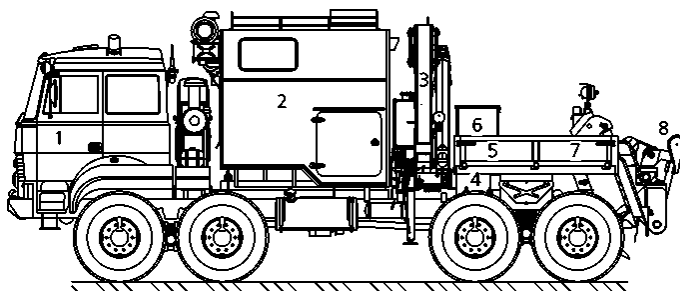
Рис. 3.10 Машина ремонтно-эвакуационная колесная легкая РЭМ-К:
