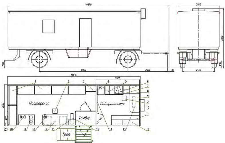
Рис. 3.43 Расположение оборудования в кузове-фургоне мастерской:
