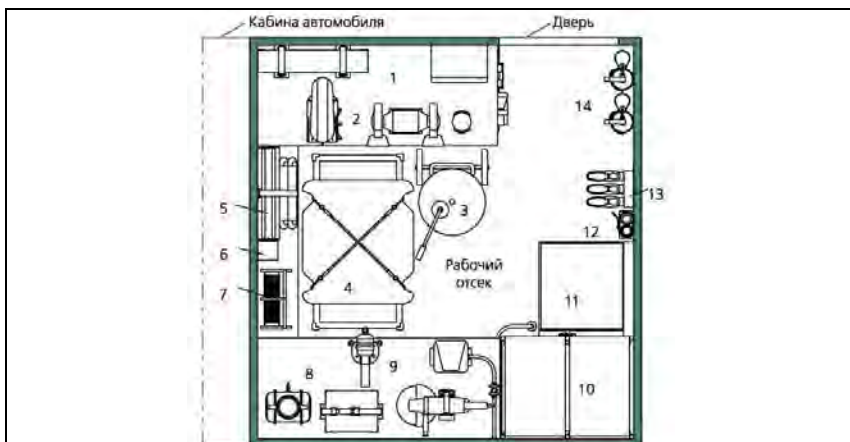
Рис. 3.11 Расположение основного оборудования в кузове-фургоне в РЭМ-К: 1 - верстак правый с ящиками для инструментов; 2 - оборудование верстака правого; 3 - установка С223-1; 4 - контейнер; 5 - стол выносной, стул складной (2 шт); 6 - навесной ящик (для документов); 7 - катушка шланговая КШУ; 8 - верстак левый с ящиками для инструментов; 9 - оборудование верстака левого; 10 - шкафы; 11 - сиденье; 12 - гамак подвесной; 13 - аптечка; 14 - огнетушители
