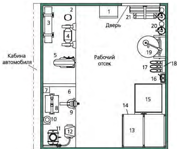
Рис. 3.14 Расположение основного оборудования в кузове-фургоне в РЭМ-КС:
