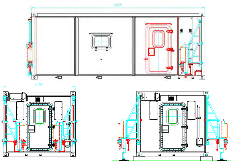
Рис. 4.4 Съемный кузов-контейнер постоянного объема
