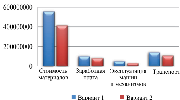
Рис. 5. Сметная стоимость циклической продольной навдвижки по вариантам
