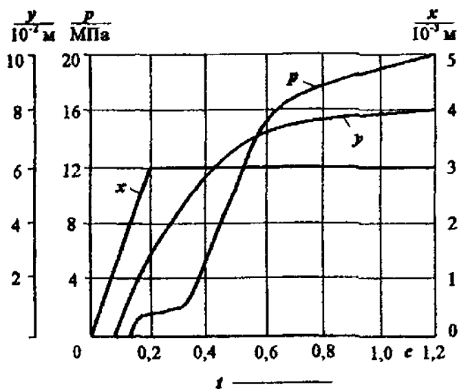
Рисунок 3.2 – Динамические характеристики гидропривода
