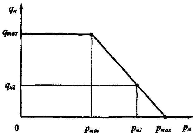
Рисунок 3.1 – Статическая характеристика авторегулируемого насоса
