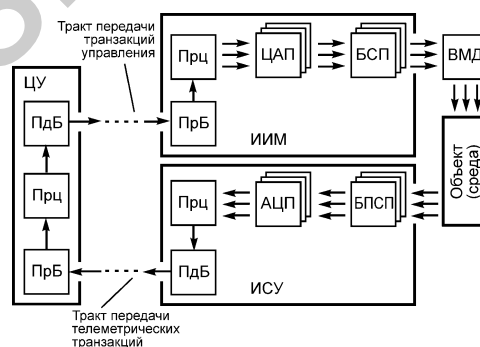
Рис. 1. Структурно-функциональная схема интеллектуальной мехатронной системы с дистанционным взаимодействием компонентов
