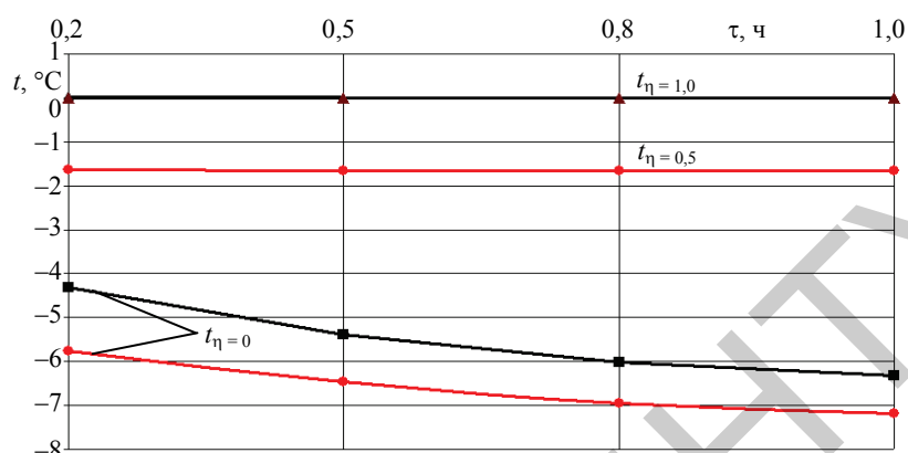
Рис. 2. Зависимости t = f(\tau, R, \eta) : —■— при R = 1,0 \text{ м}^2 \cdot \text{К/Вт} ; —●— при R = 2,0 \text{ м}^2 \cdot \text{К/Вт} ; —▲— — рассчитанные значения температур t_{\eta=0,5} при R = 1,0 \text{ м}^2 \cdot \text{К/Вт} малы и графики t_{\eta=0,5} при R = 1,0 \text{ м}^2 \cdot \text{К/Вт} и t_{\eta=1,0} при R = 1,0 \text{ м}^2 \cdot \text{К/Вт} и R = 2,0 \text{ м}^2 \cdot \text{К/Вт} фактически совпадают с осью координат
