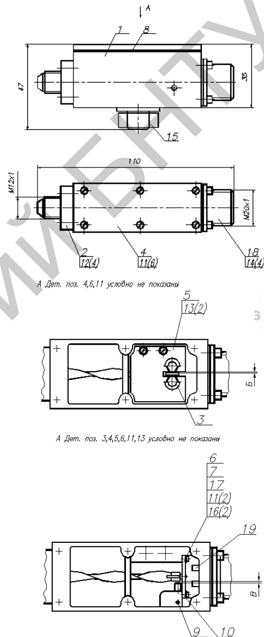
Рисунок 2 – Конструкция датчика
