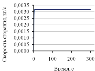
Рисунок 2 – Зависимость массовой скорости сгорания топлива от времени в источнике пожара мощностью 150 кВт
