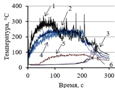
Рисунок 4 – Зависимости температуры воздуха от времени в центре закрытой комнаты на высоте 0,1 (3, 5, 6) и 2,4 м (1, 2, 4) при пожаре с источником на полу (4,5), на высоте 0,7 (2, 6) и 1,7 м (1, 3)
