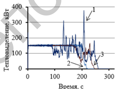
Рисунок 3 – Зависимости тепловыделения от времени при пожаре мощностью 150 кВт с источником на полу (2), на высоте 0,7 м (3) и 1,7 м (1) в закрытой комнате
