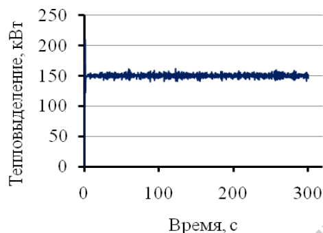
Рисунок 5 – Зависимость тепловыделения от времени при пожаре с источником на высоте 1,7 м в комнате с вентиляцией
