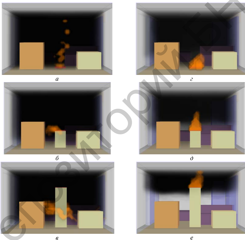
Рисунок 6 – Картины на 200-й секунде пожаров в закрытой комнате (а, б, в) и в комнате с естественной вентиляцией (г, д, е) с источником мощностью 150 кВт на полу (а, г), на высоте 0,7 (б, д) и 1,7 м (в, е)
