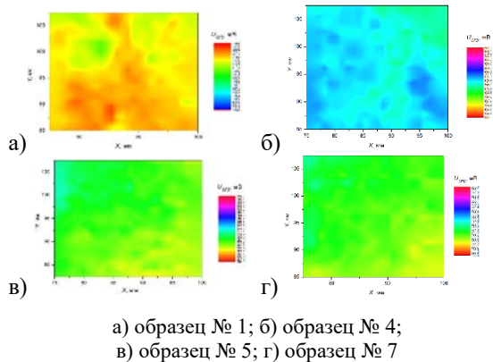
Рисунок 1 – Пространственное распределение РВЭ поверхности оптических деталей высшего класса чистоты
