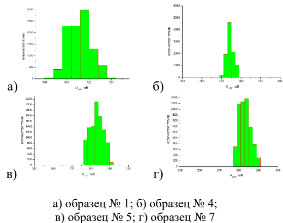
Рисунок 2 – Гистограммы распределения значений РВЭ
