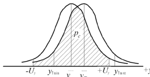
Рисунок 1 – Графическая интерпретация показателя p_c (probability coincidence)
