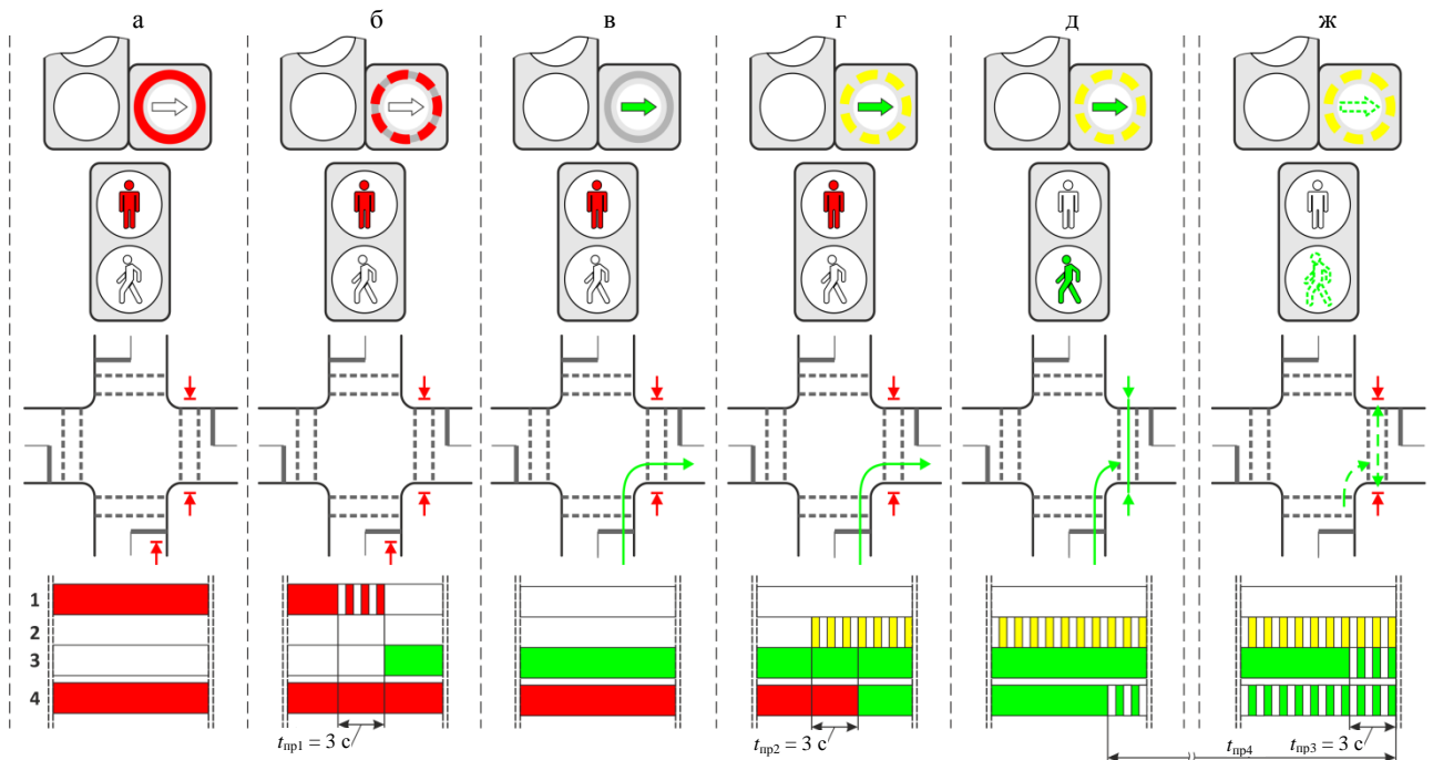
Рис. 3. Оповещение водителей о наличии дополнительной секции, о переходном интервале и приоритете:
