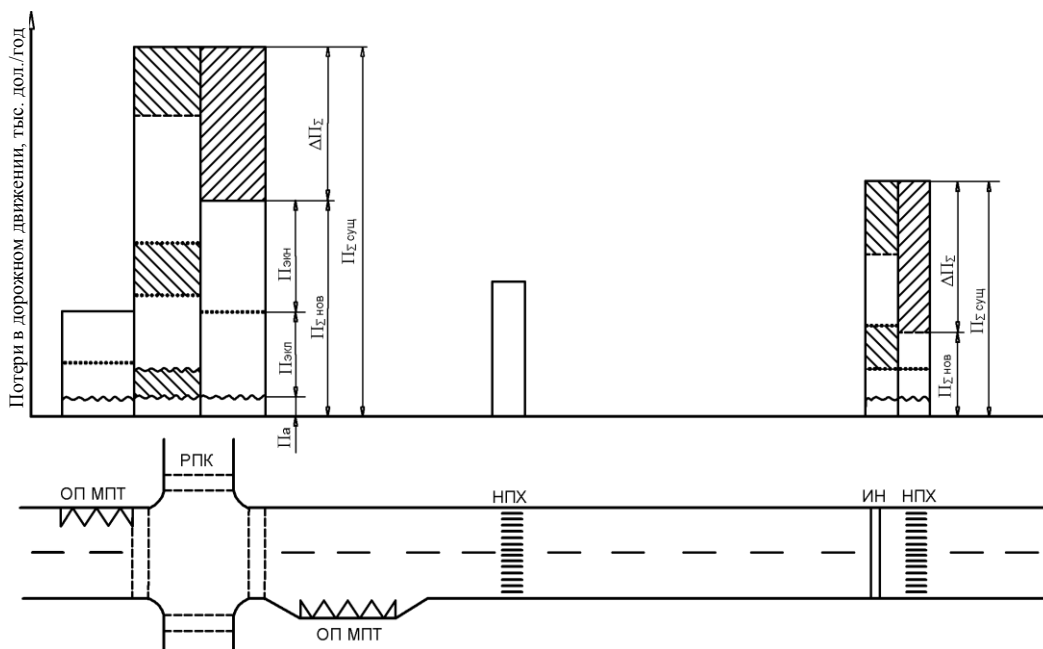
Рис. 7. Линейный график очаговых потерь в дорожном движении на городской улице: ~~~~ – аварийные потери;
