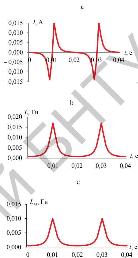
Рис. 7. Временные диаграммы тока (а), индуктивности (б) и взаимной индуктивности (с) возвратно-поступательного электрического генератора
