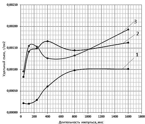
Рисунок 1 – Зависимости съема материала образца из алюминия технического АД1 от длительности импульсов и плотности тока
