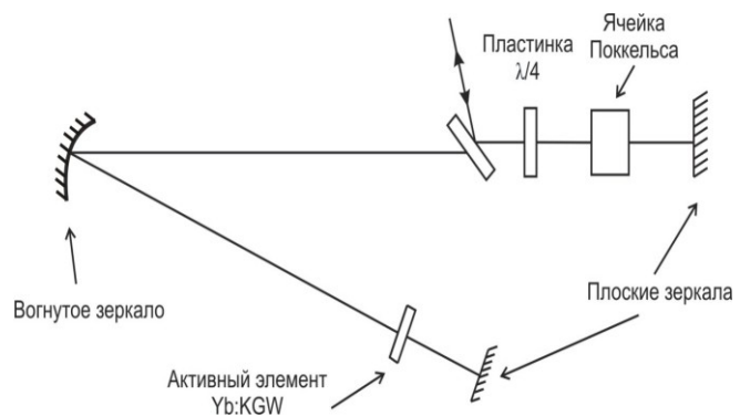
Рисунок 5 – Схема резонатора усилителя
