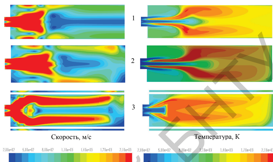
Рис. 5. Поля скорости и температуры: 1, 2 – топка с аксиальным и боковым выходом соответственно; 3 – топка водотрубно-дымогарного котла
