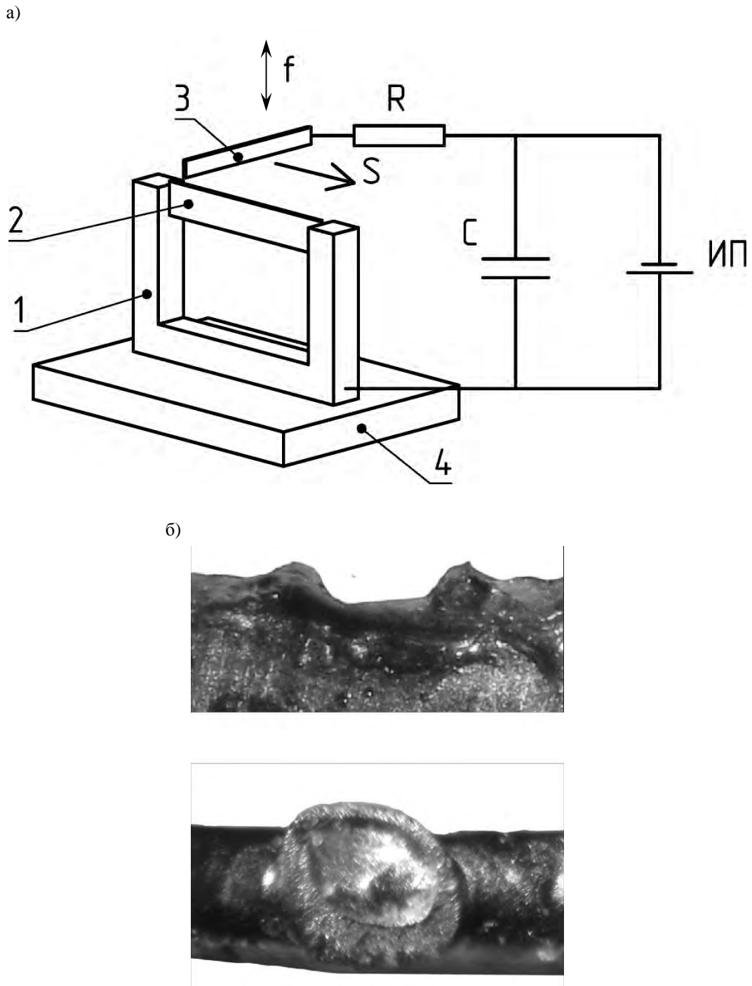
Рис. 1. Схема электроэрозионного модифицирования поверхности штрипсы (а); лунка, полученная на поверхности штрипсы (б)
