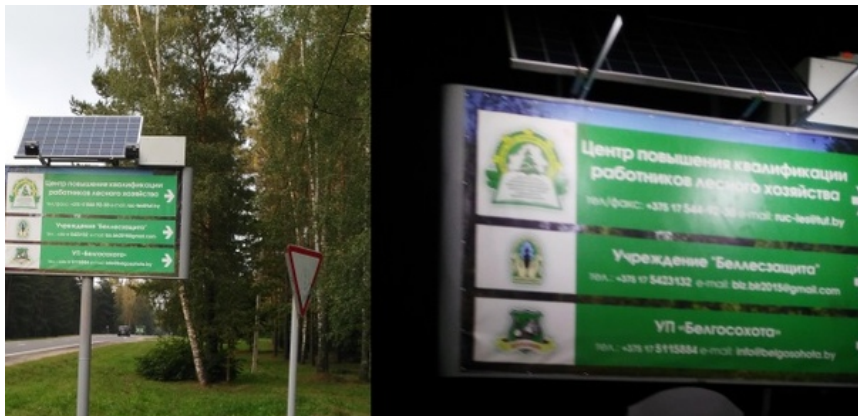
Рисунок 2 – Комплект оборудования для подсветки баннера размером 2.5*1.5м. Установлен в этом году в Минском районе. В этом случае, достаточно 4 светильников мощностью 10Вт и напряжением 24В.
