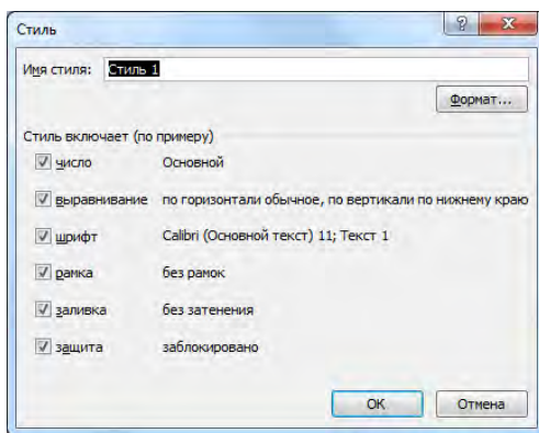
Рисунок 25 – Стиль форматирования
