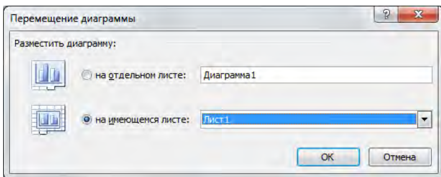
Рисунок 71 – Расположение диаграммы
