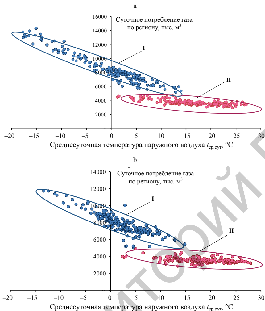
Рис. 5. Поле соответствия суточного потребления газа в регионе среднесуточной температуре на годовом интервале времени за 2014 г. (а) и 2015 г. (б):
