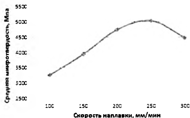
Рисунок 4 – Зависимость средней микротвердости в валике из бронзы ПГ-19М-01 от скорости наплавки
