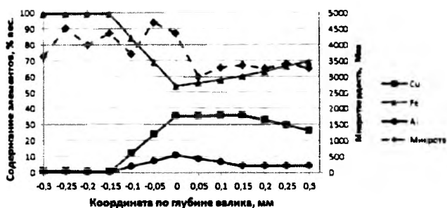
Рисунок 2 – Распределение элементов и микротвердости по глубине валика из бронзы ПГ-19М-01, нанесенного лазерной наплавкой при скорости наплавки 100 мм/мин и дистанции наплавки 12 мм
