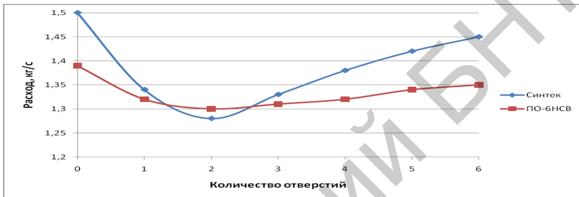
Рисунок 12 – Зависимость расхода огнетушащего вещества от количества отверстий для газонасыщения в оросителе с диаметром узкого сечения эжектора D = 9,6 мм
