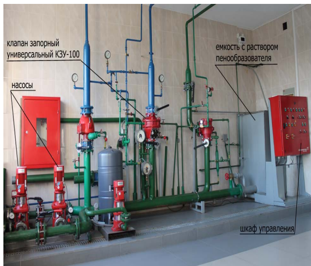
Рисунок 1 – Фотография лабораторной установки для проведения исследований
