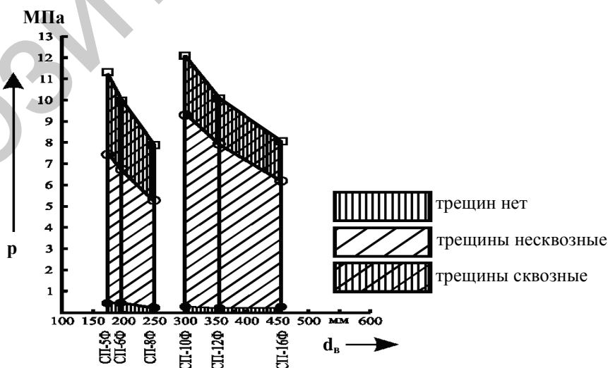
Рисунок 3 – Характер изменения предельных давлений при трех стадиях работы фильтров с внутренними диаметрами d_b
