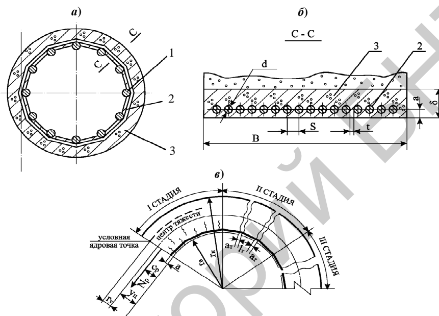
а – поперечный разрез; б – продольный разрез; в – расчетная схема; 1 – стержни каркаса фильтра; 2 – проволочная навивка; 3 – цементированная гравийная обсыпка Рисунок 1 – Схема заcolmатированного каркасно-стержневого фильтра
