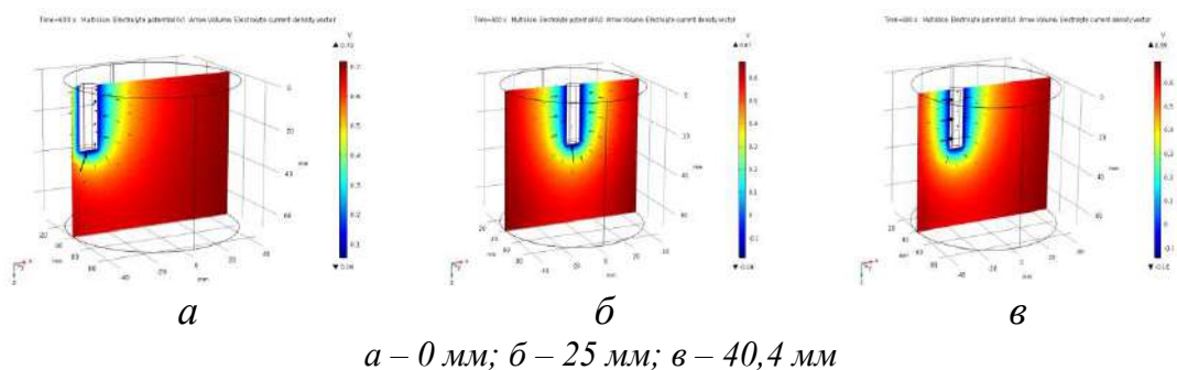
Рисунок 2 – Конфигурация электрического потенциала электролита при смещении осей электродов
