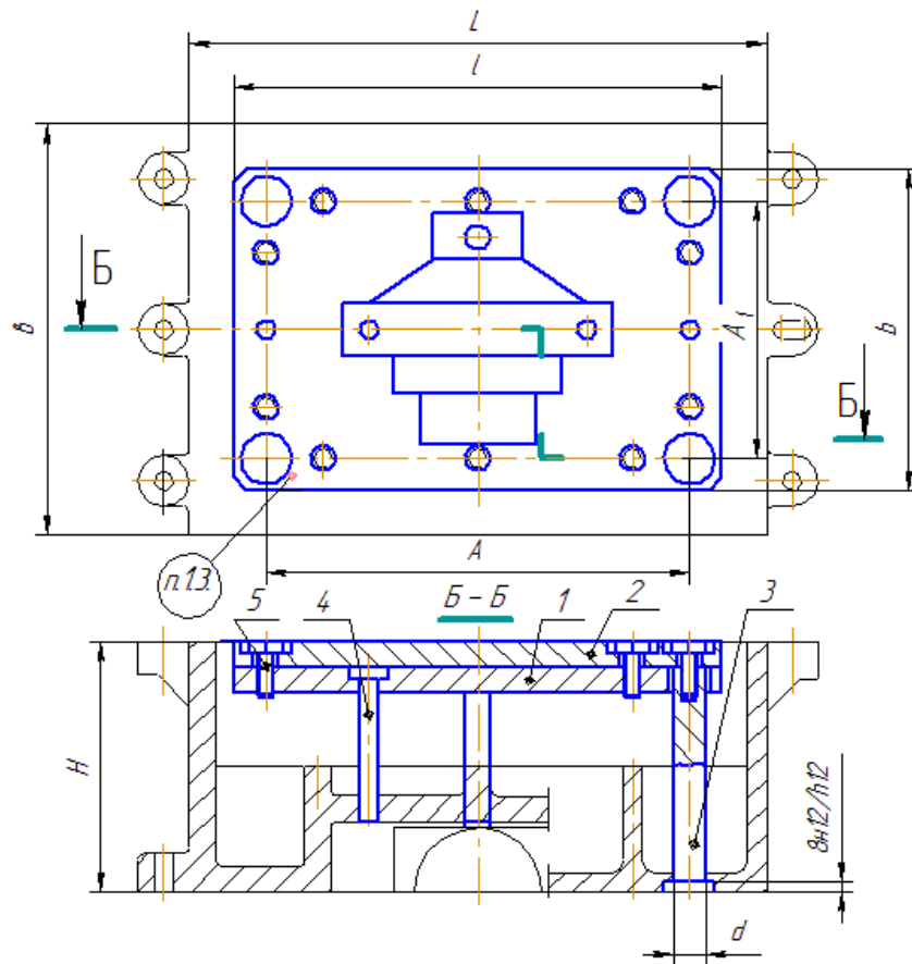
Рис. 3.31. Приспособление для выталкивания отливок из металлической формы с параллельным разъемом 1 – Плита выталкивателей, 2 – Плита опорная, 3 – Контртолкатель, 4 – Выталкиватель, 5 – Винт
