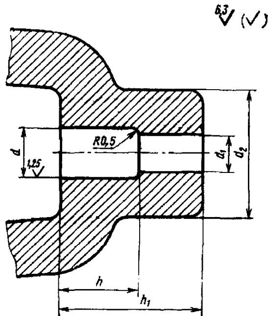
Рис.3.27 Эскиз выполнения отверстий под пружинные выталкиватели
