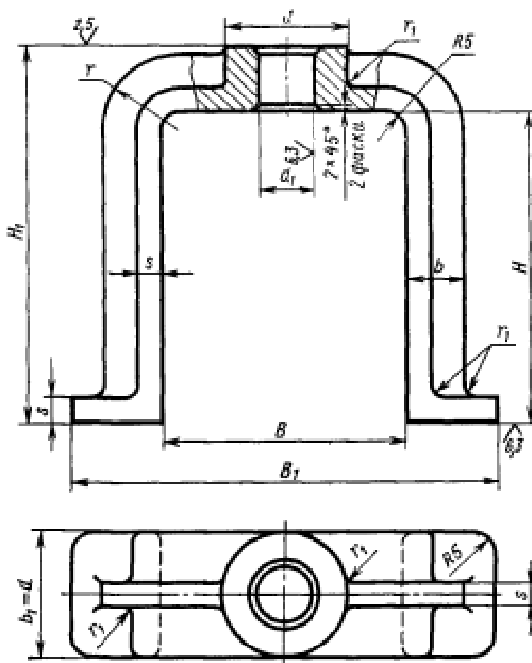
Рис.3.36. Скоба винтового приспособления для удаления стержней
