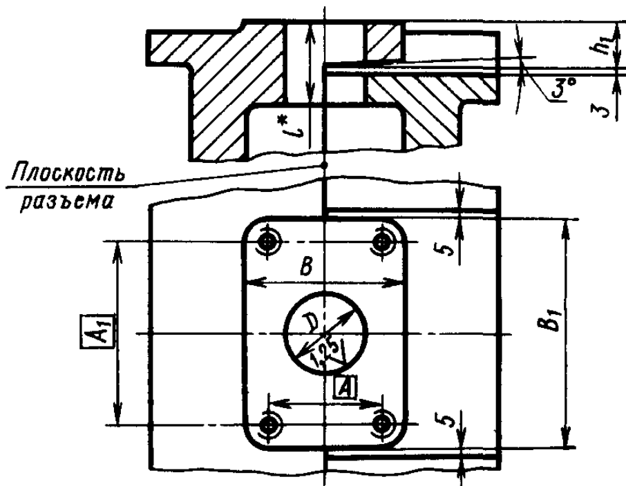
Рис3.54. Конструкция платиков для установки пневматического приспособления
