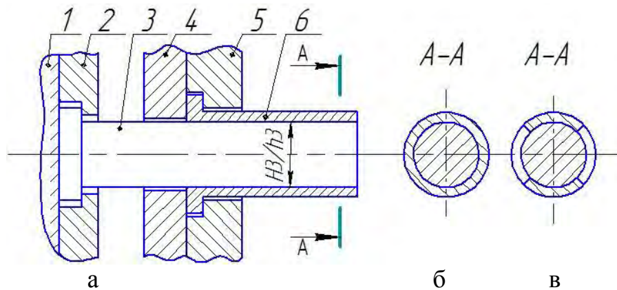
Рис.3.29 Пример крепления трубчатого сегментного выталкивателя
