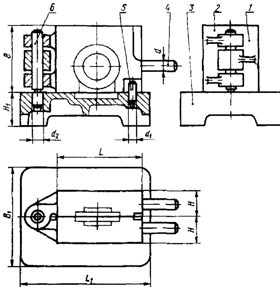
Рис.3.10. Конструкция створчатых металлических форм
