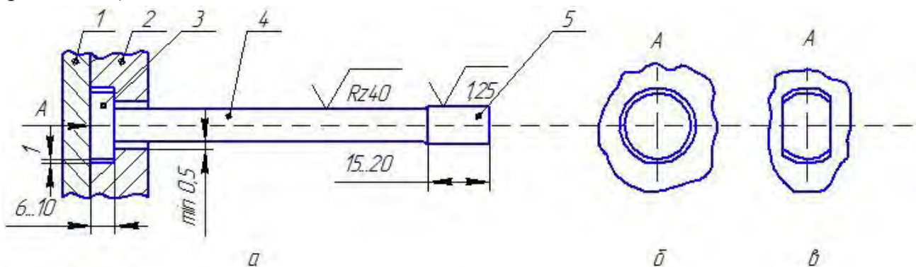
Рис. 3.28. Пример крепления штифтового выталкивателя для механизированных кокилей
