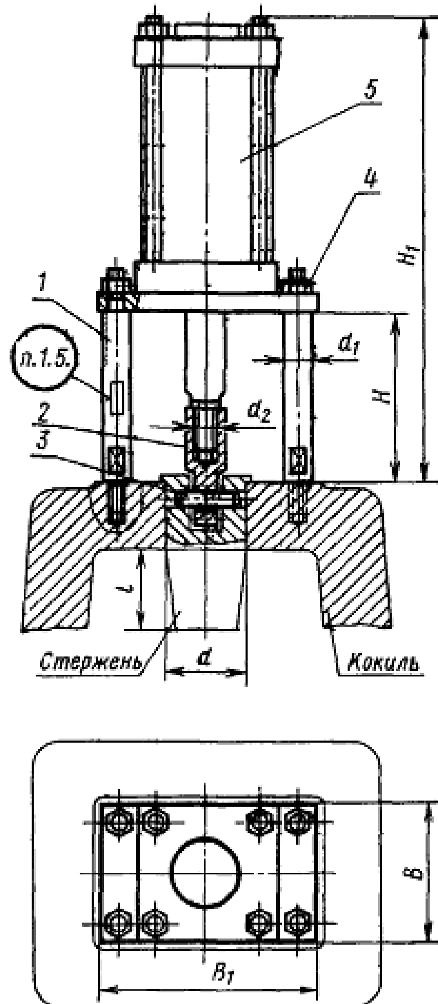
Рис. 3.52. Приспособление для удаления стержней пневматическое
