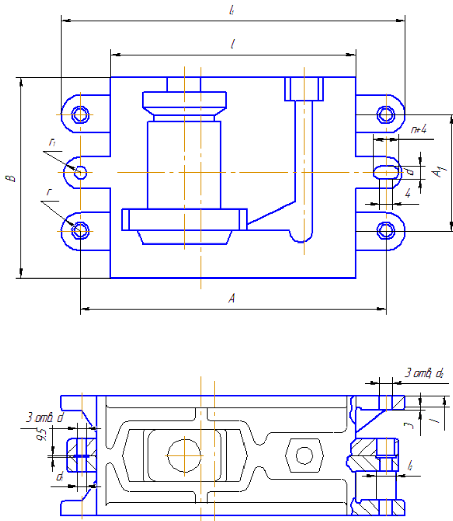
Рис.3.15.Металлическая форма с параллельным разъемом
