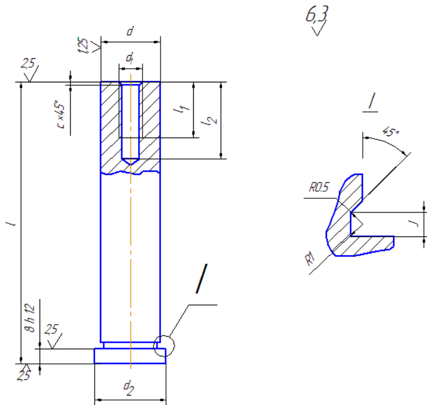
Рис.3.34 Контролкатель механизма выталкивания
