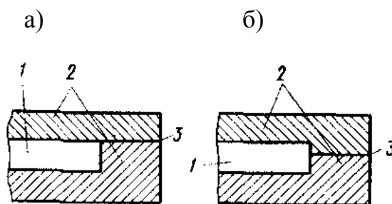
Рис.1.6. Расположение поверхности разъема кокиля по отношению к стенке отливки а – неправильное; б – правильное; 1–отливка; 2–кокиль; 3–поверхность разъема
