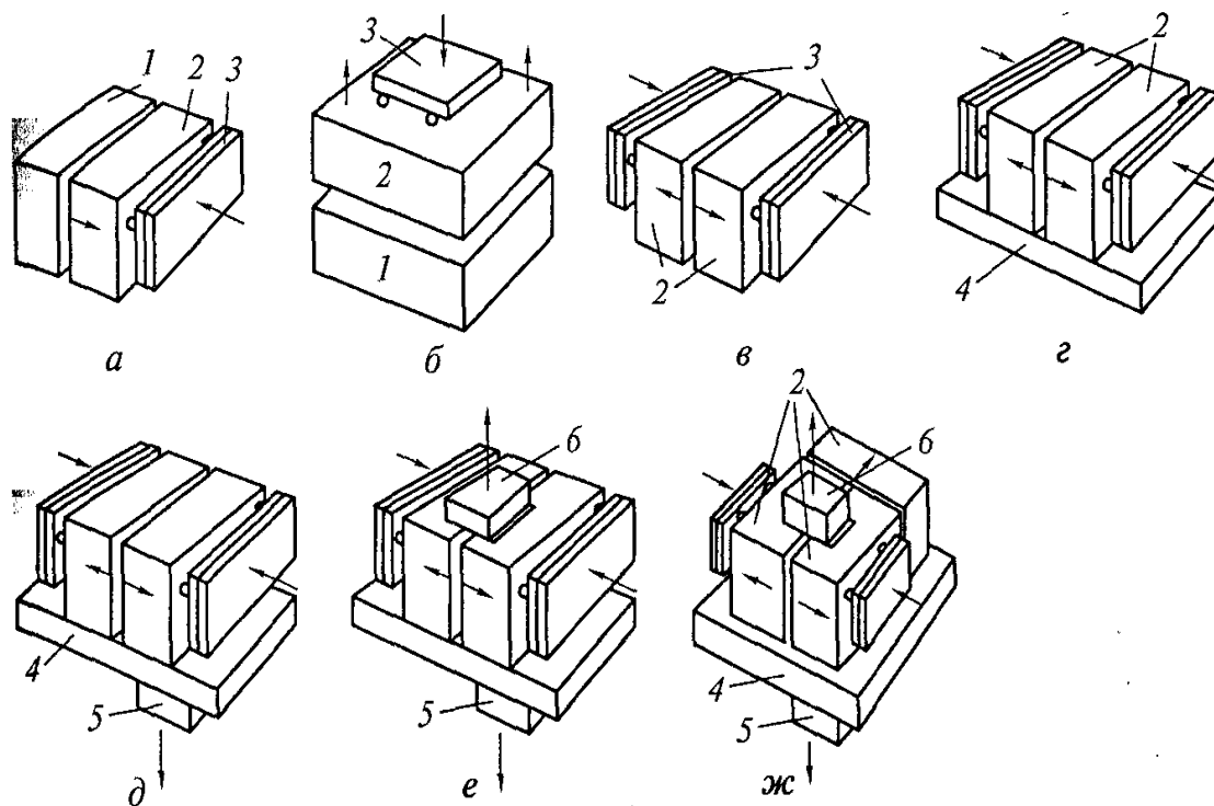
Рис. 3.4. Типы кокилей для универсальных кокильных машин.
