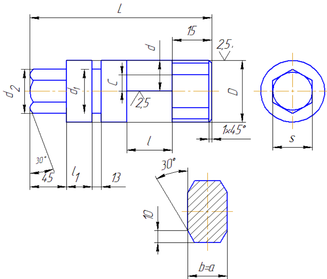
Рис.3.42. Эксцентрик для удаления стержней
