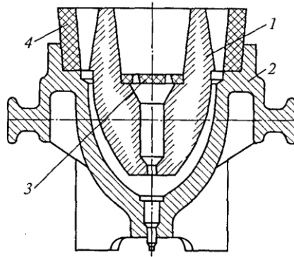
Рис. 3.1 Вытряхной кокиль:
