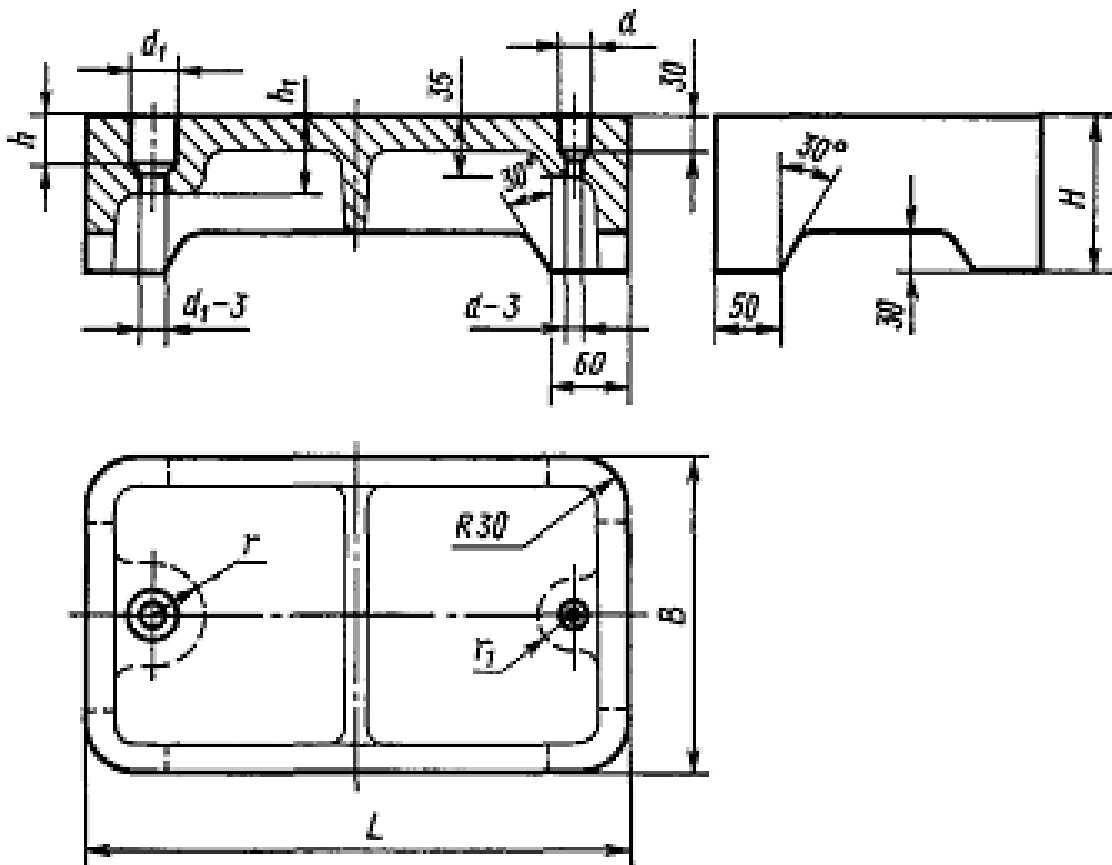
Рис.3.13. Плита основания створчатого кокиля
