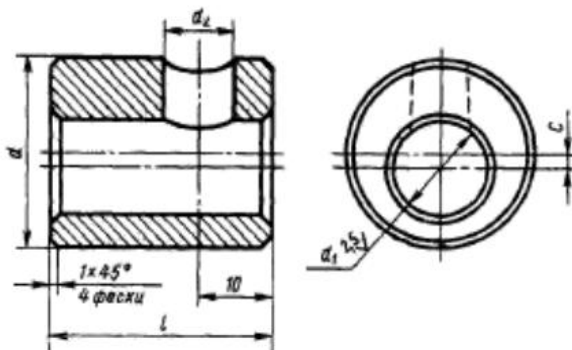
Рис.3.20. Конструкция эксцентриковой втулки
