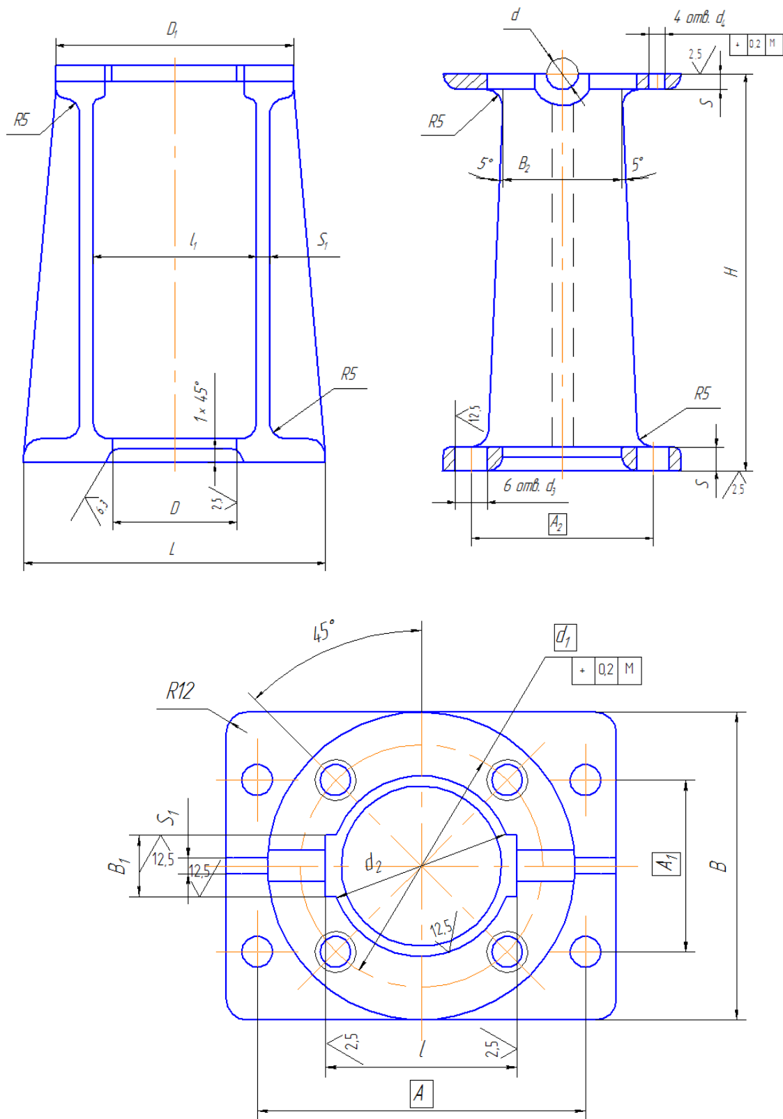
Рис. 3.47. Конструкция стойки гидравлического приспособления для удаления стержней
