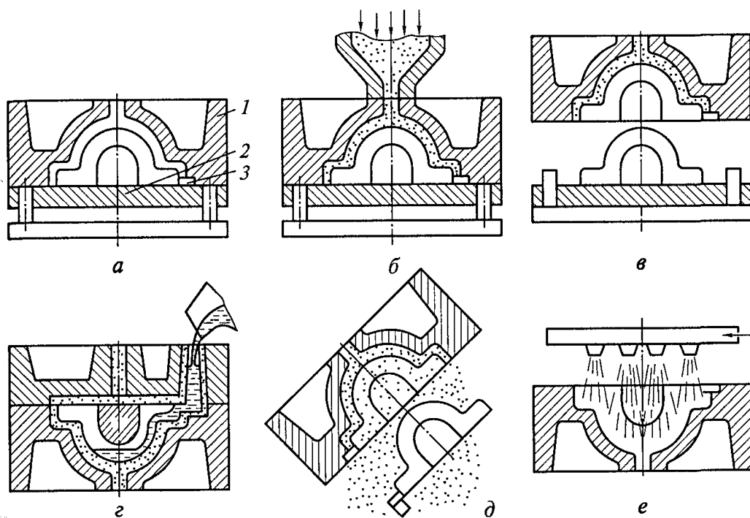
Рис.5.1. Последовательность изготовления отливки в облицованном кокиле: а – нагрев кокиля; б – нанесение облицовочного слоя (стрелками показано направление подачи смеси); в – удаление модели; г – сборка и заливка кокиля; д – удаление отливки; е – очистка кокиля; 1 – кокиль; 2 – модельная плита; 3 – зазор
