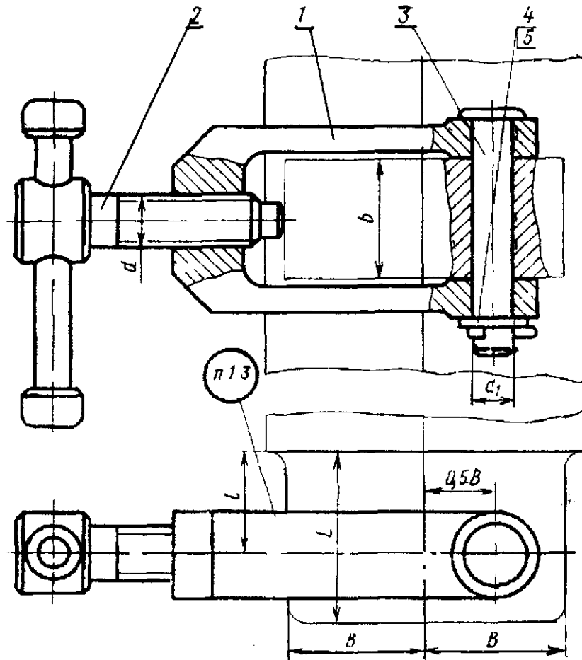
Рис.3.17. Винтовой замок для скрепления створчатых кокилей
