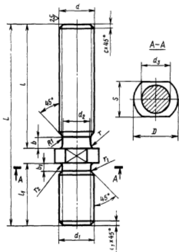
Рис. 3.37. Винт приспособления для удаления стержней
