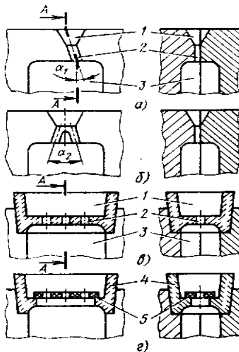
Рис. 2.2 Схемы литниковых систем для заливки сверху кокилей с вертикальным разъемом
