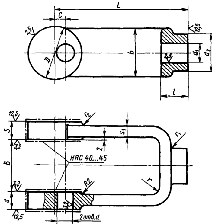
Рис.3.40. Скоба эксцентрикового приспособления
