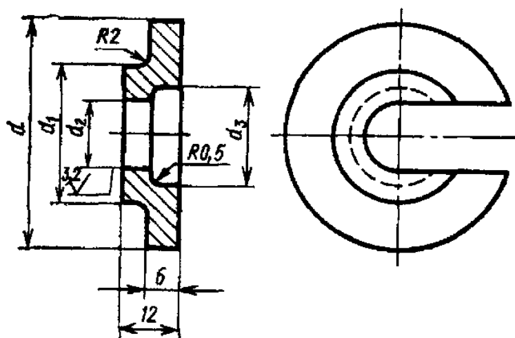
Рис. 3.25 Конструкция фиксирующей шайбы
