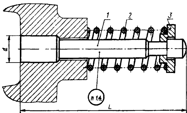
Рис. 3.23. Конструкция пружинного механизма выталкивания 1 – выталкиватель; 2 – пружина; 3 – шайба
