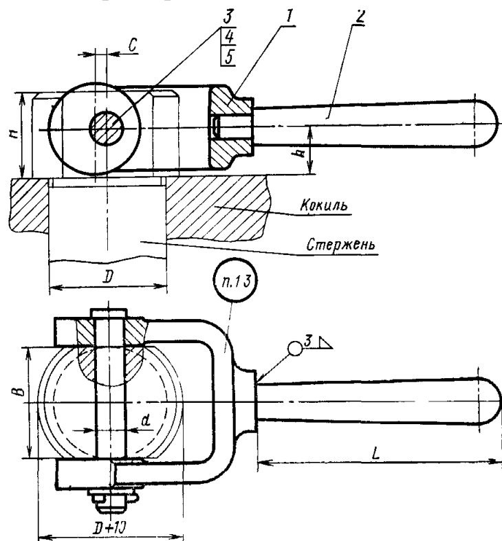
Рис. 3.39. Приспособление для удаления стержней эксцентриковой скобой
