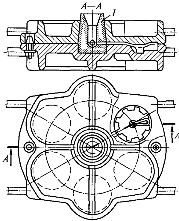
Рис.3.2. Кокиль с горизонтальной плоскостью разъема:
