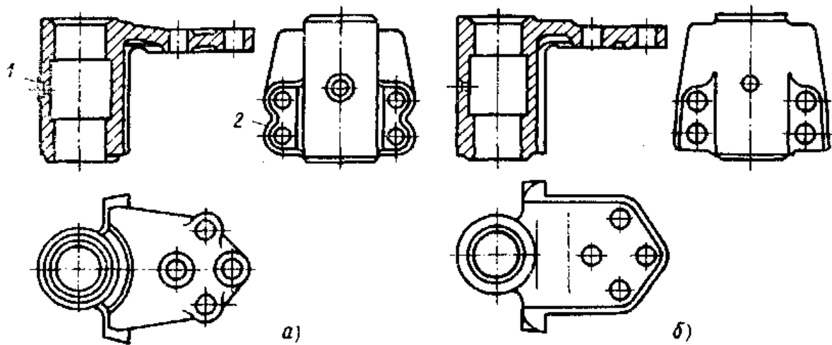
Рис.1.3 Отливка стального кронштейна а) нетехнологично; б) технологично
