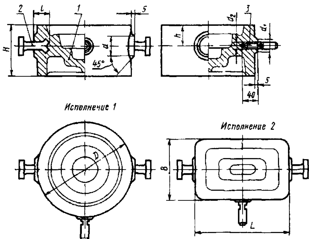
Рис.3.9. Вытряхной кокиль 1 – металлическая форма; 2 – цапфа; 3 –ручка ввертная.
