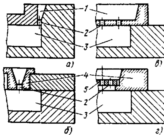
Рис. 2.1 Схемы литниковых систем для заливки сверху кокилей с горизонтальным разъемом и литниковой чашей и питателем:
