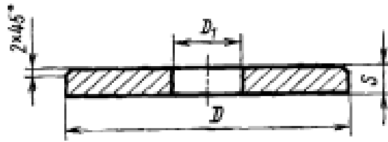
Рис.3.59 Конструкция и размеры опорной шайбы приспособления для удаления стержней
