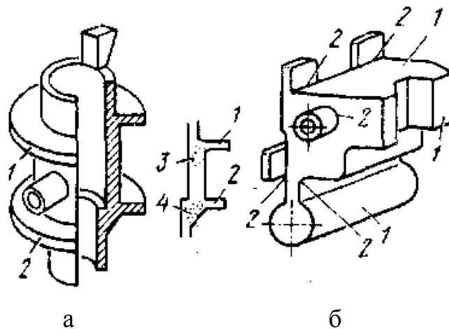
Рис. 1.5. Нетехнологичные конструкции отливок втулки (а) и корпуса (б) из алюминиевого сплава
