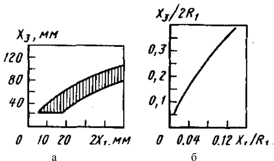
Рис.3.5. Графики для выбора толщин стенок плоских (а) и цилиндрических (б) кокилей
