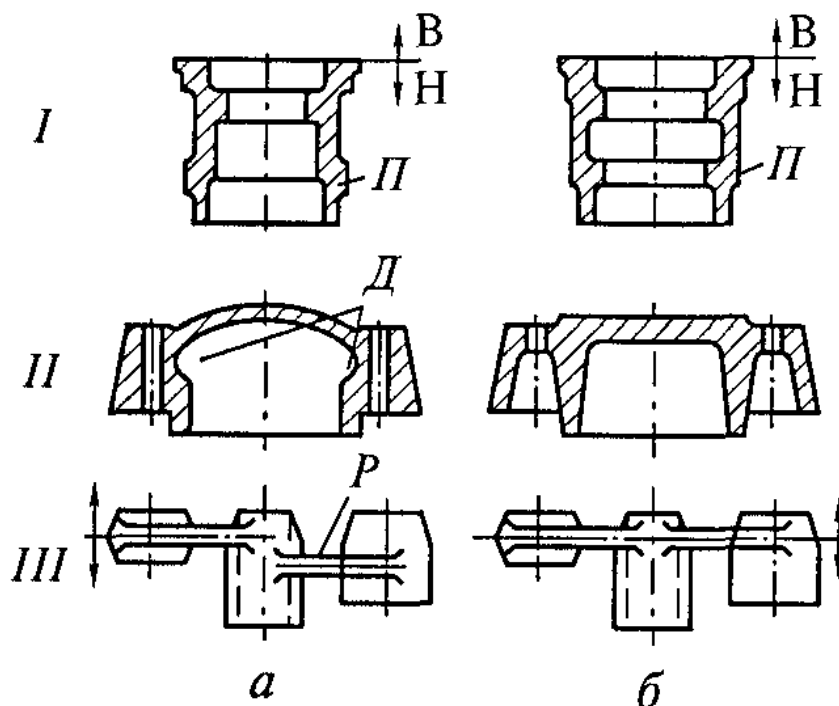
Рис. 1.2. Конструкции кокильных отливок: а – неправильные (1– 111); б – правильные (1– 111); П – поясок; Д – поднутрение; Р – ребро; В, Н – верх и низ линии разъема кокиля
