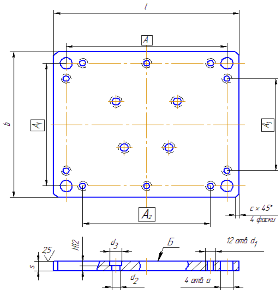
Рис.3.32 Конструкция плиты выталкивателей
