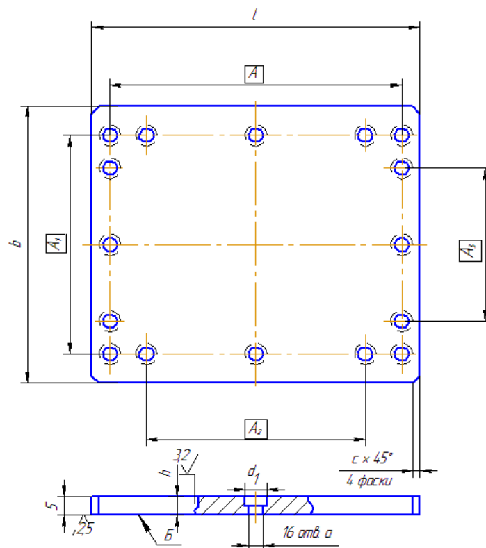
Рис. 3.33. Конструкция опорной плиты
