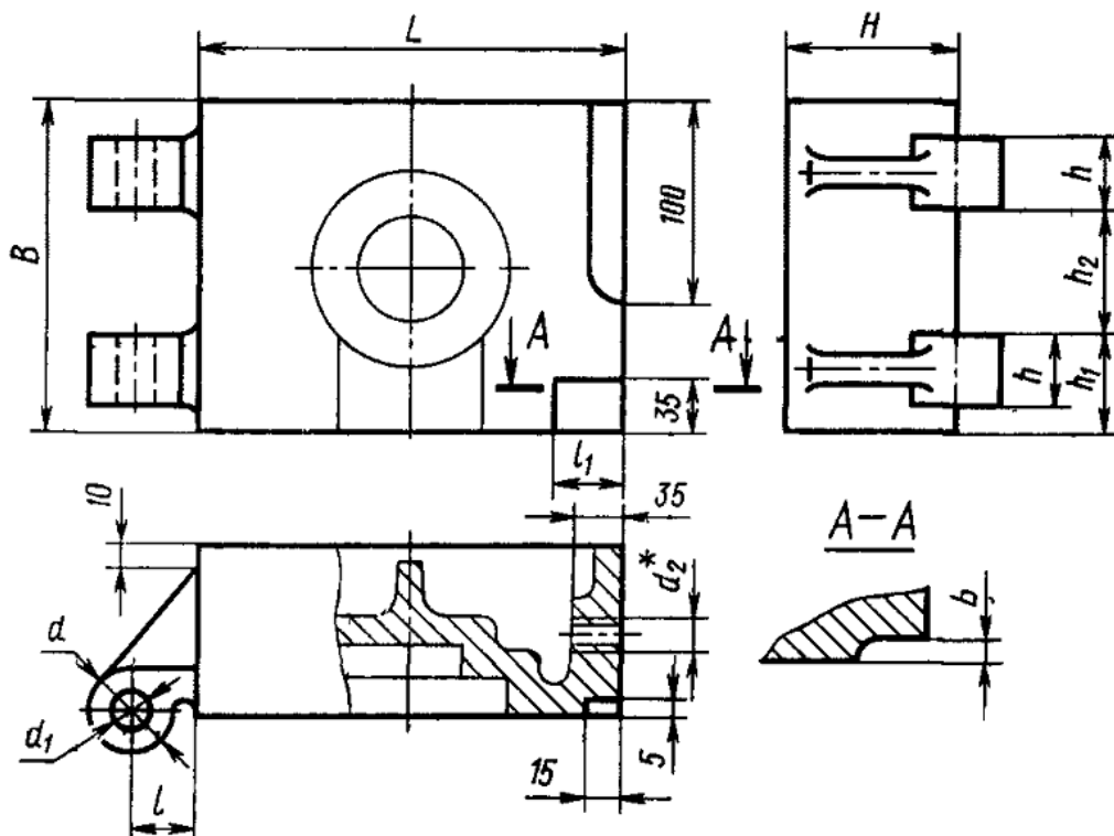
Рис.3.12. Конструкция правой полуформы кокиля
