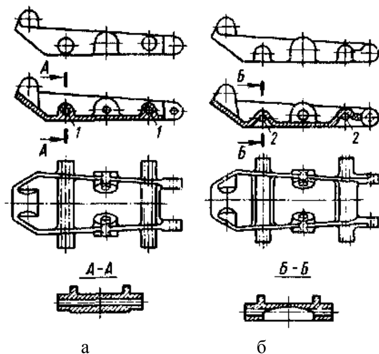
Рис. 1.4.Конструкция отливки из алюминиевого сплава: а – нетехнологичная; б–технологичная
