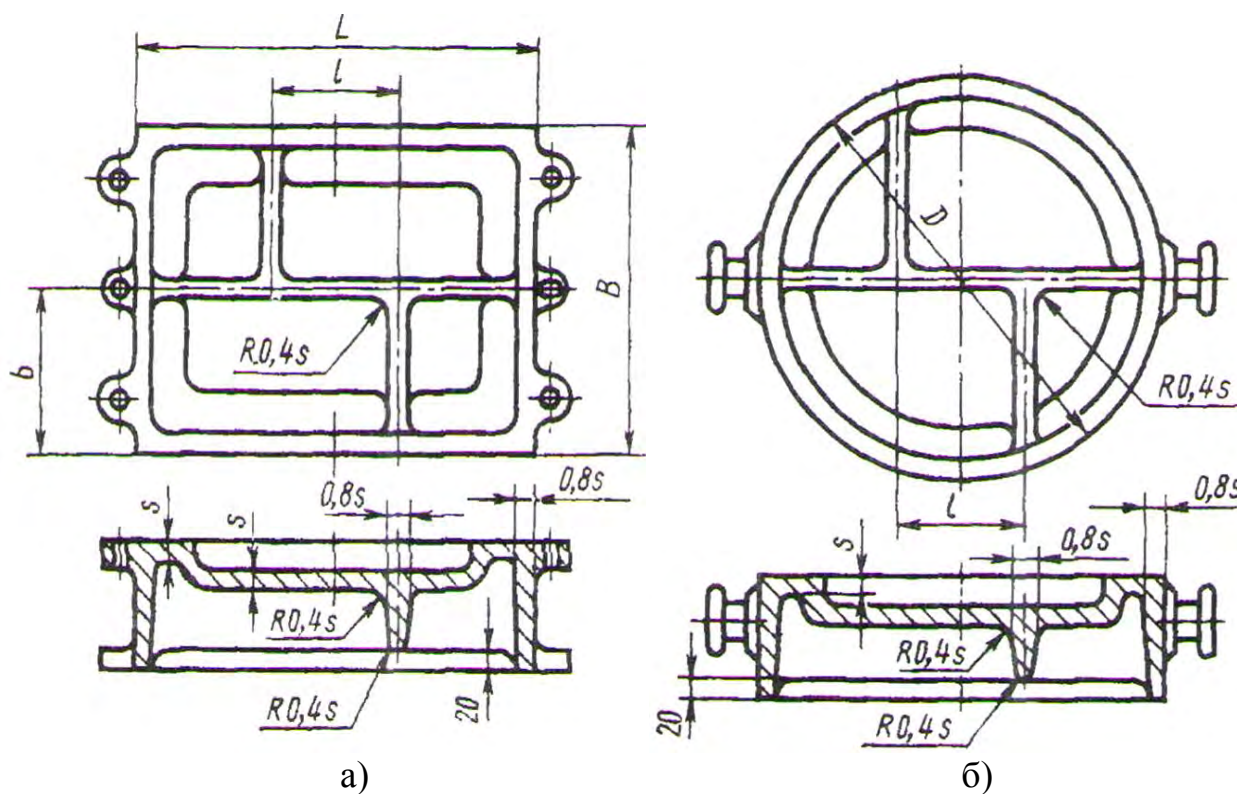
Рис.3.7. Расположение ребер жесткости на прямоугольных (а) и круглых (б) кокилях размером 400 x 320 и 500 x 400; L , B и D – длина, ширина и диаметр кокиля s – толщина стенки металлической формы
