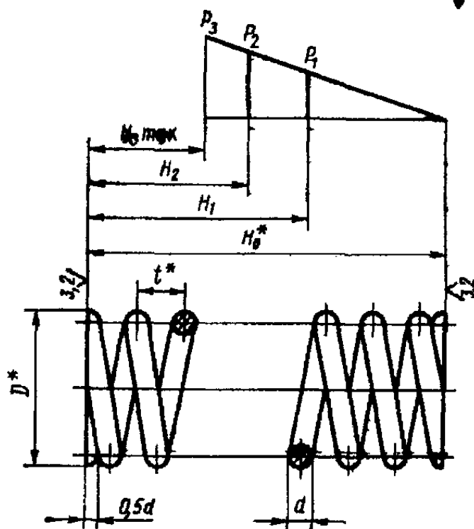
Рис.3.26. Пружина механизма выгалкивани
