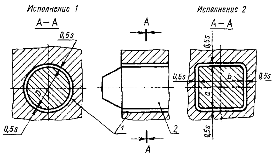
Рис.3.30. Примеры расположения зазоров между направляющими металлическими стержнями и металлической формой
