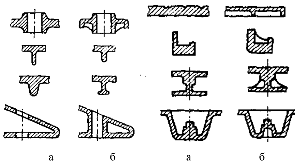
Рис. 1.1. Конструктивные элементы отливок: а – нетехнологичные; б – технологичные
