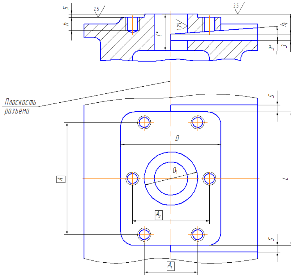
Рис. 3.51. Конструкция платика для установки гидравлического приспособления
