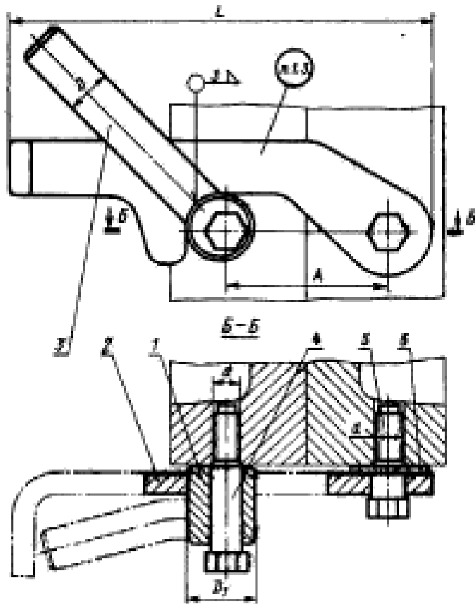
Рис.3.19.Конструкция эксцентриковых замков
