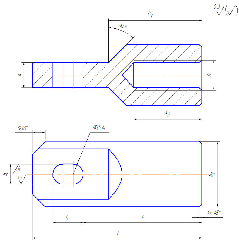
Рис. 3.49. Конструкция тяги гидравлического приспособления для удаления стержней
