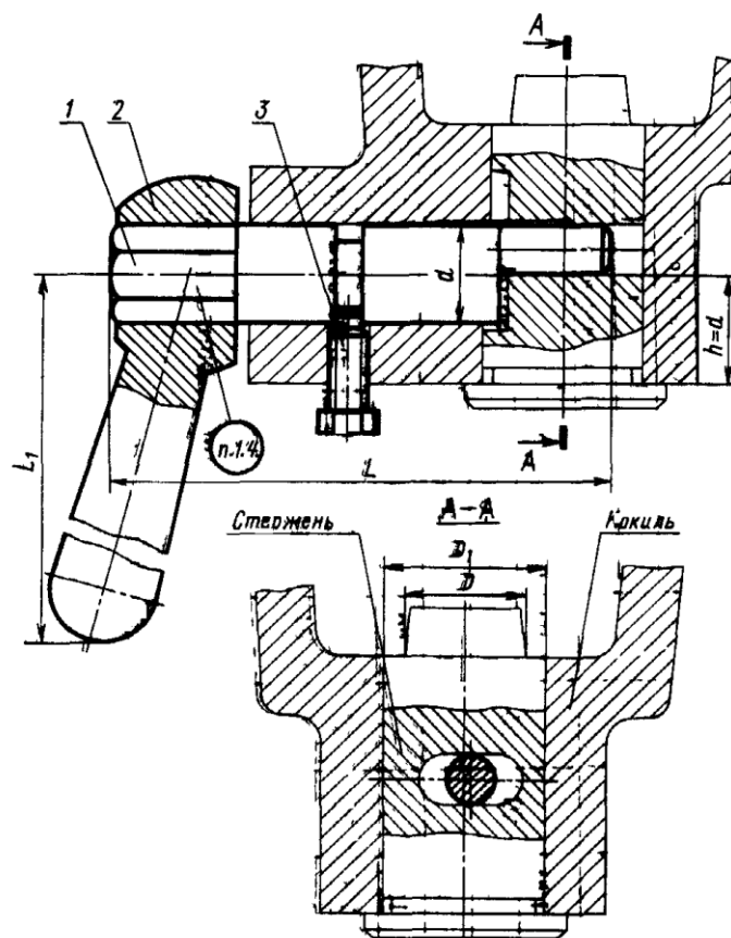
Рис. 3.44 Конструкция приспособления для удаления стержней консольным эксцентриком.
