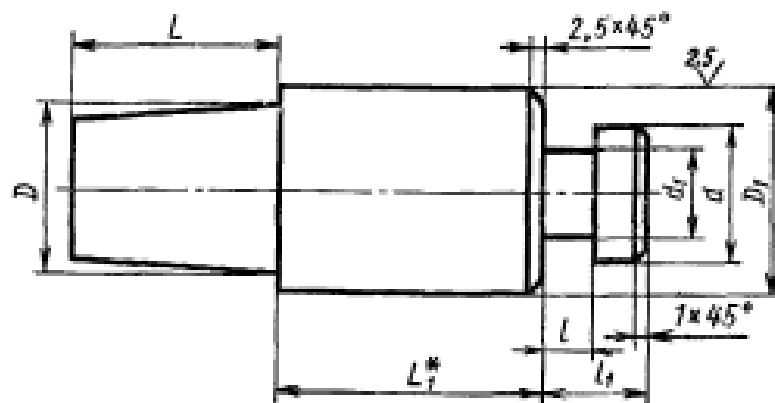
Рис.3.60 Конструкция стержней, удаляемых речными приспособлениями
