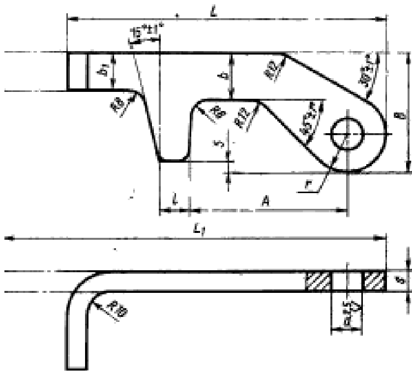
Рис.3.21. Конструкция замка
