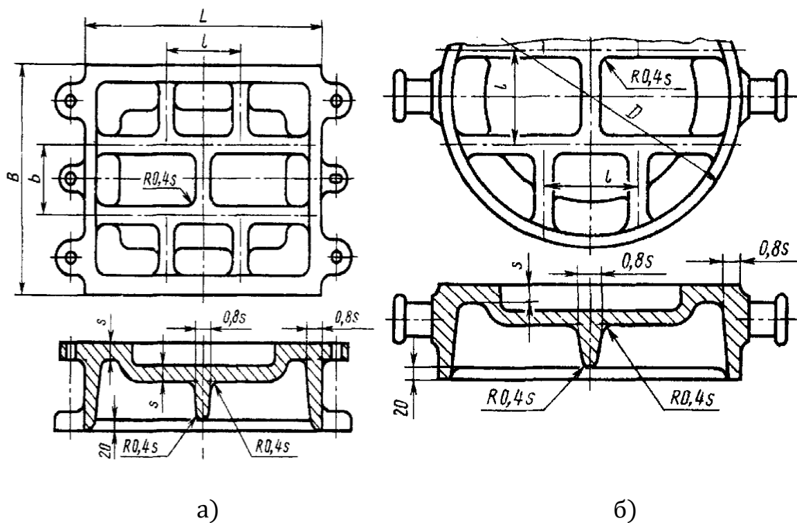
Рис.3.8. Расположение ребер жесткости на прямоугольных (а) и круглых (б) кокилях размером 600 x 500 и выше s – толщина стенки металлической формы L , B и D – длина, ширина и диаметр кокиля
