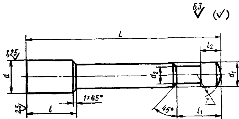
Рис. 3.24 Конструкция выталкивателя
