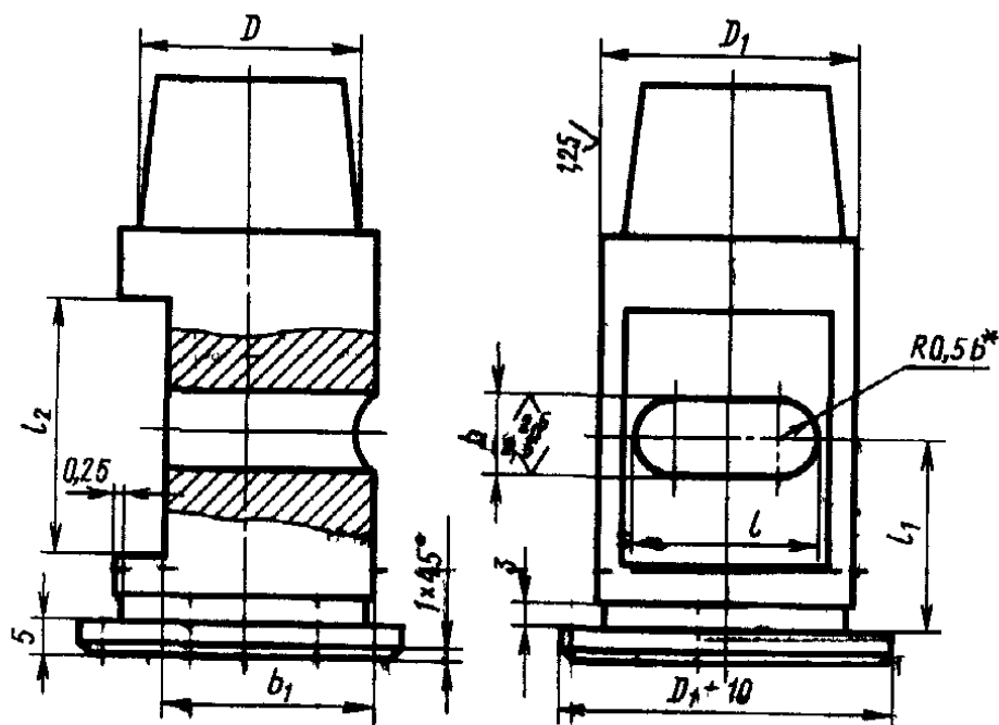
Рис.3.43. Конструкция стержней, удаляемых эксцентриковыми приспособлениями
