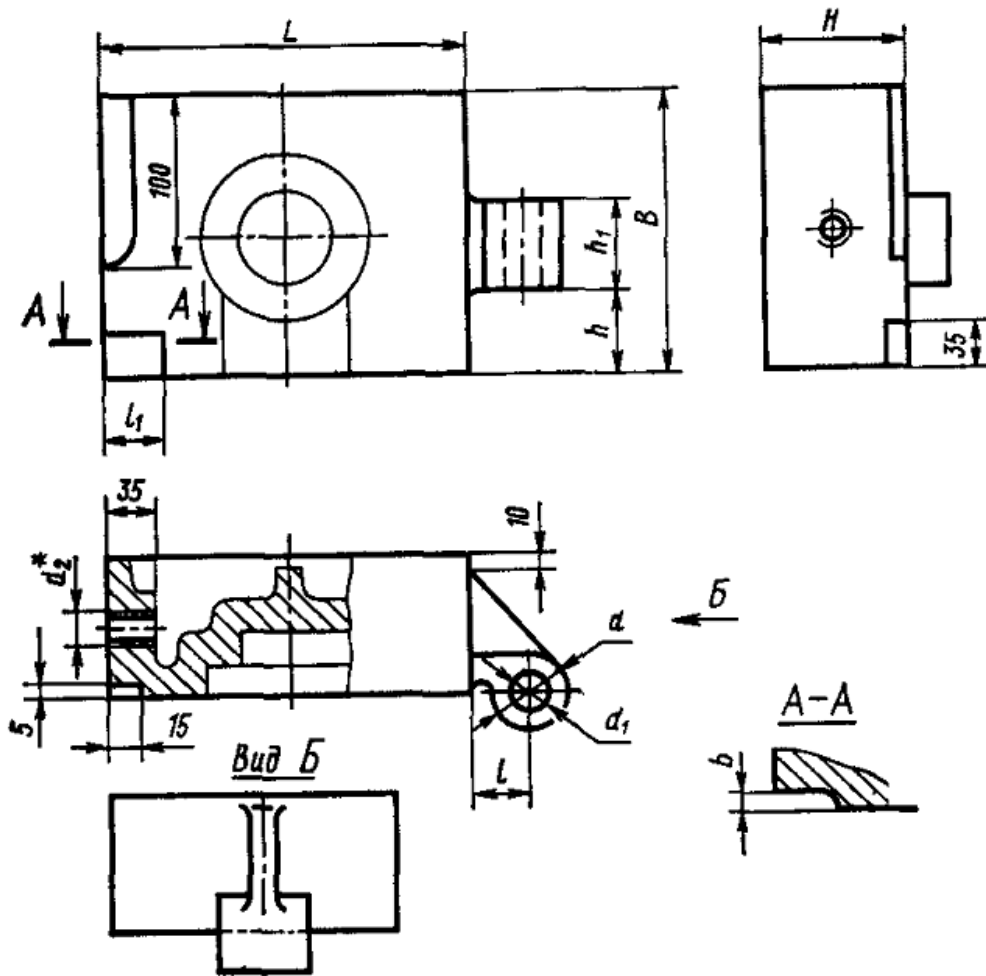
Рис. 3.11. Конструкция левой полуформы кокиля
