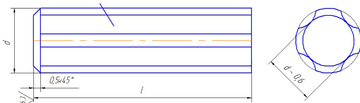
Рис 2.9 Пробки вентиляционные проходные
