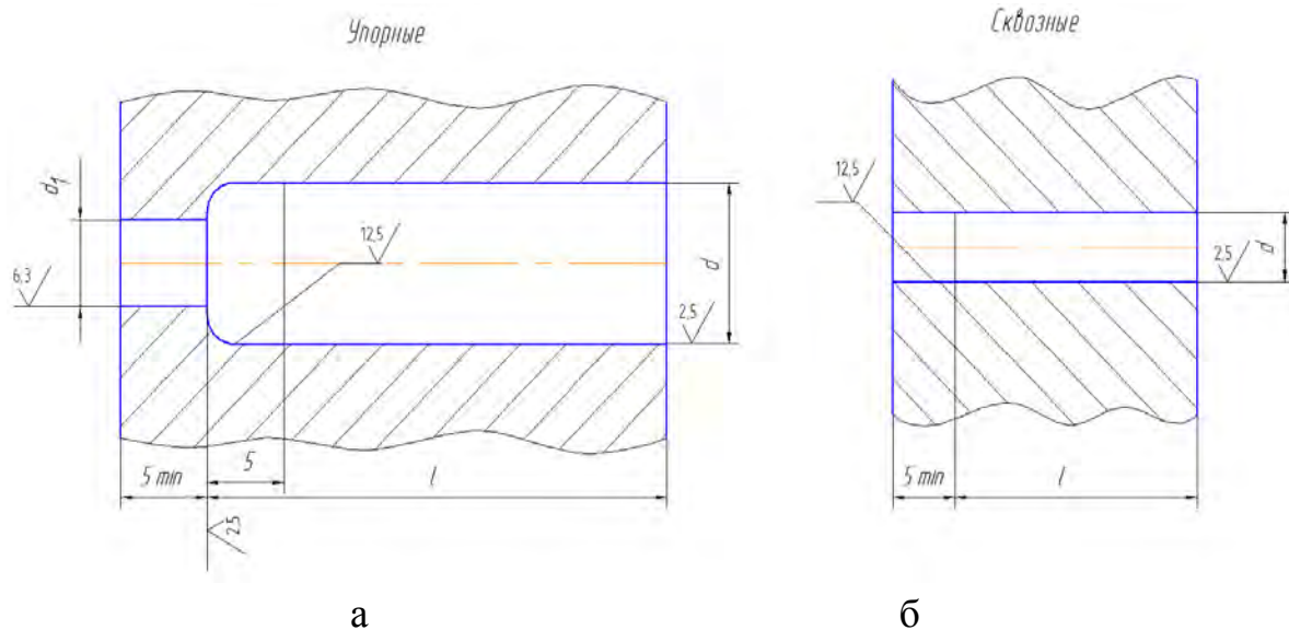
Рис.2.7. Конструкция отверстий для установки вентиляционных пробок а – отверстия для упорных пробок; б – отверстия под проходные пробки
