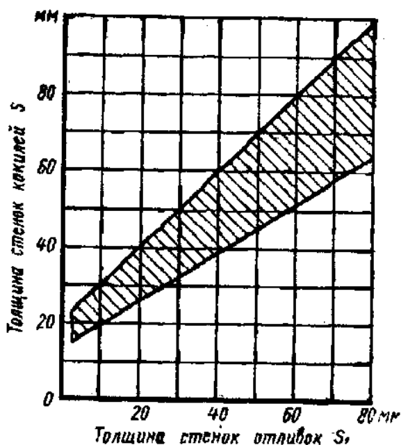
Рис.3.6. График для выбора толщины стенки кокиля
