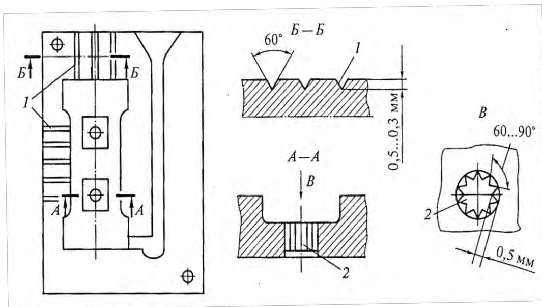
Рис.2.6 Вентиляционная система кокиля:
