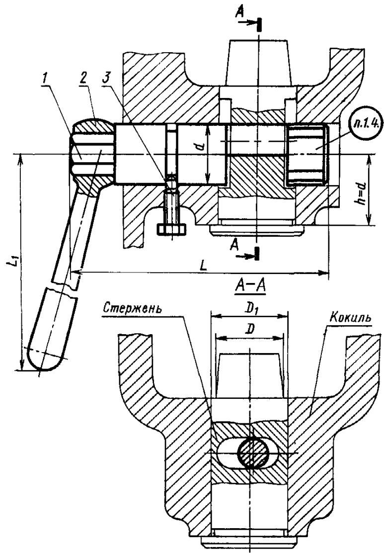
Рис. 3.41. Приспособление для удаления стержней эксцентриковое
