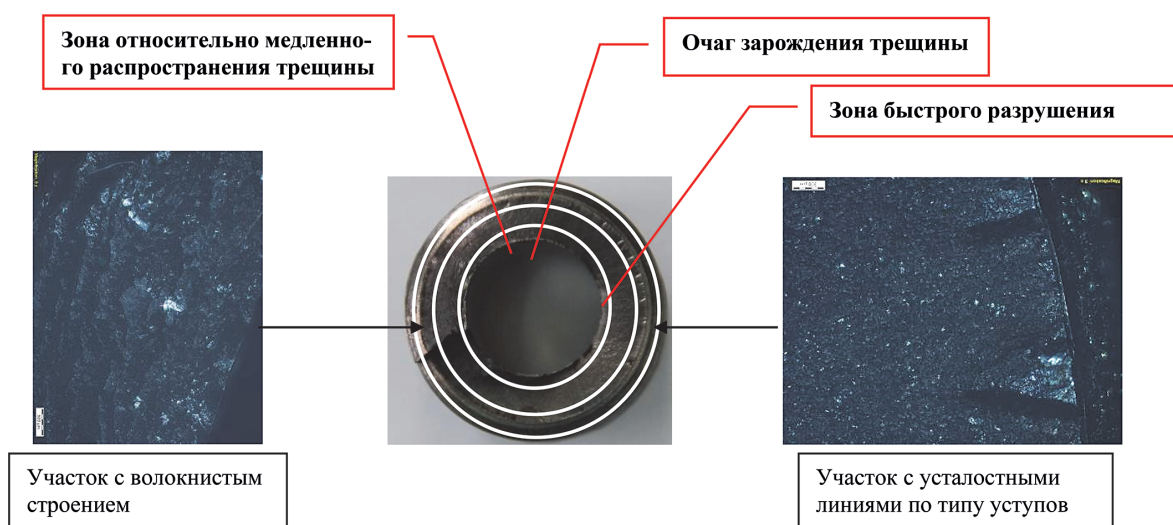
Рис. 2. Внешний вид поверхности излома с фотографиями макростроения отдельных участков. \times 50
