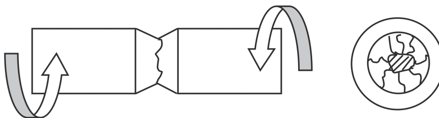
Рис. 3. Схема строения усталостного излома при кручении при высоком номинальном напряжении
