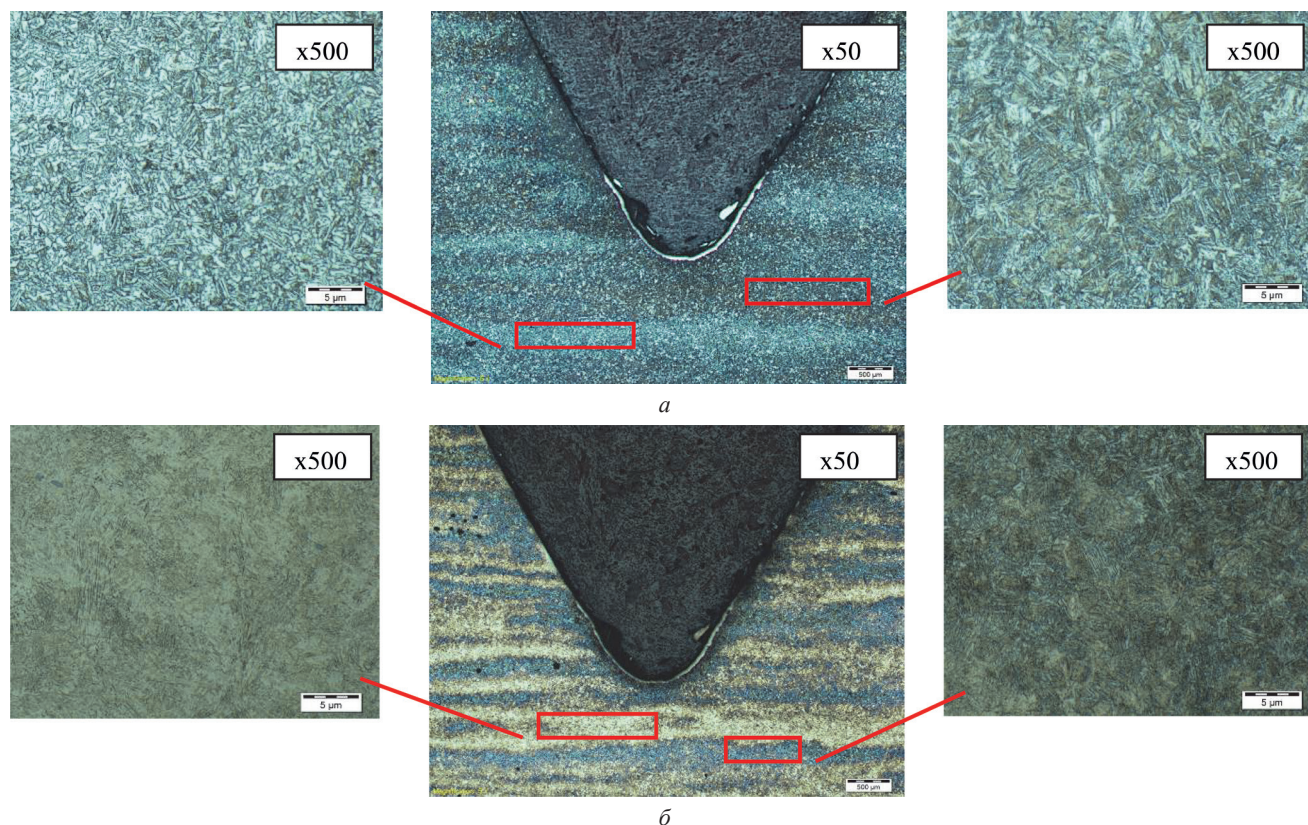
Рис. 4. Микроструктура после травления: а – реактив «Nital»; б – реактив Обергоффера
