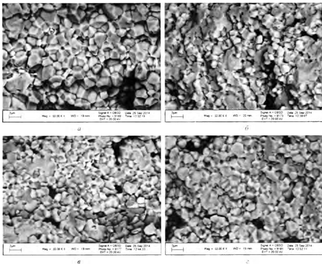
Рис. 4. Микроструктура поверхности излома керамических образцов ЦТС с различным временем механоактивации: a – без УЗВ; б – УЗВ 30 мин; г – УЗВ 60 мин; з – УЗВ 90 мин
