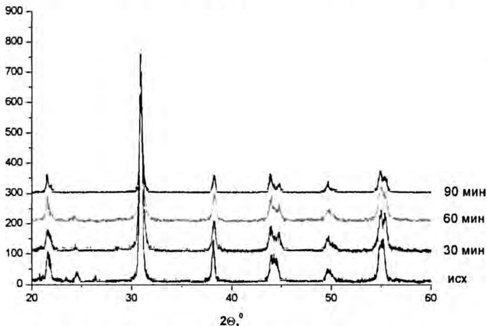
Рис. 1. Вид рентгенограмм порошков ЦТС (а) и образцов ЦТС после спекания (б) в зависимости от времени УЗВ
