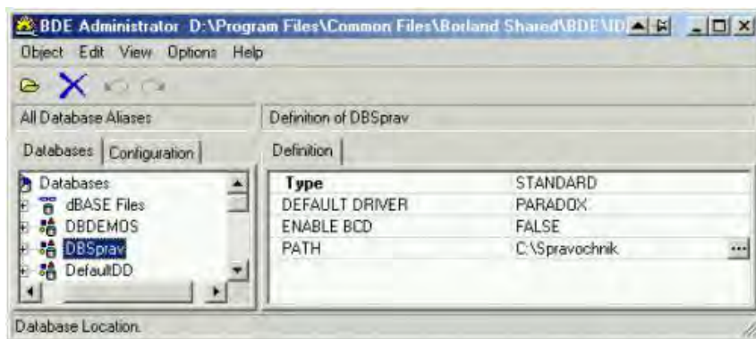
Рис. 8.4. Результат создания псевдонима
