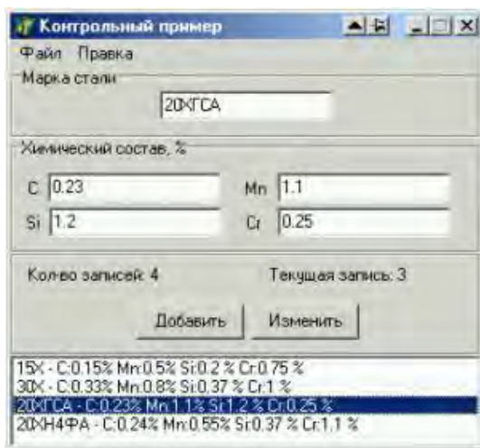
Рис. 7.4. Результат выполнения программы
