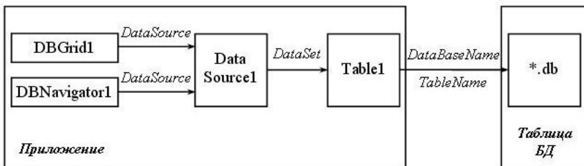
Рис. 8.3. Связь компонентов приложения и таблицы БД
