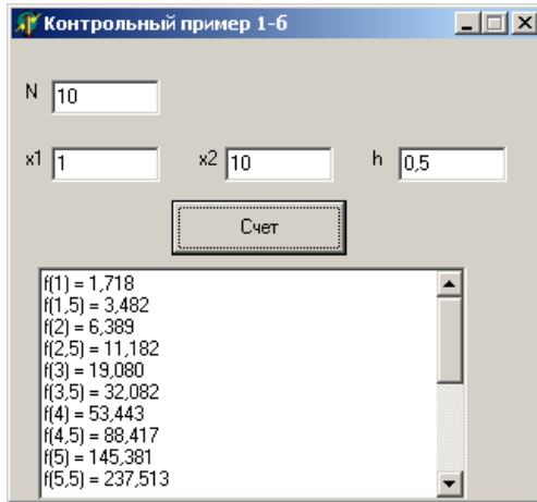
Рис. 3.1. Результат выполнения программы
