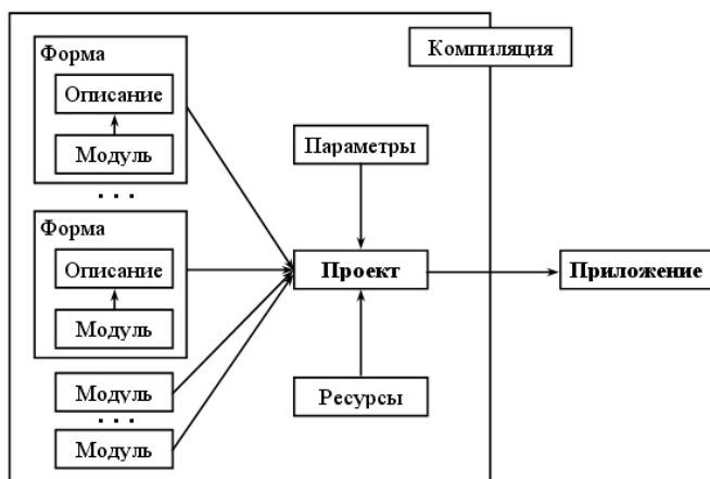
Рис. 1.2. Взаимосвязи между файлами проекта
