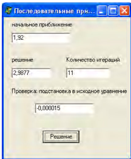
Рис. 3.2. Результат выполнения программы
