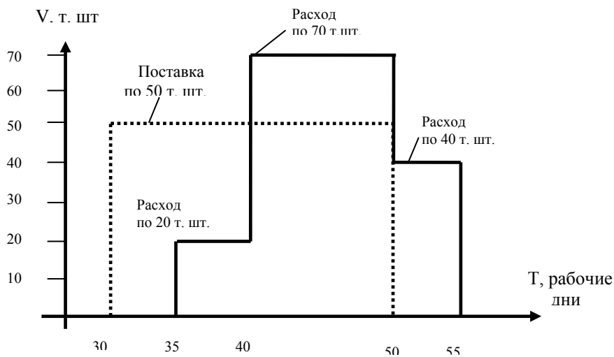
Рис. 4.2 а). Дифференциальный график при неравномерном расходовании и равномерной поставке кирпича.
