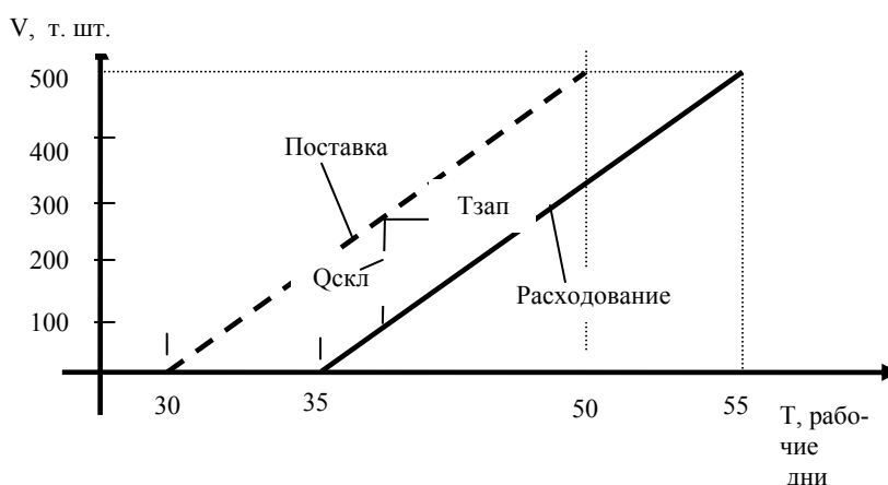
Рис. 4.3. Общий вид интегрального графика при поставке и расходе кирпича с одинаковой интенсивностью
