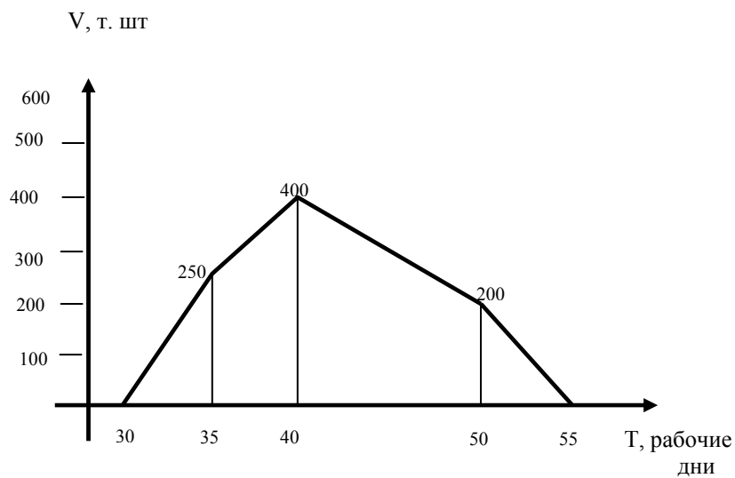
Рис. 4.2 а). Дифференциальный график при неравномерном расходовании и равномерной поставке кирпича.
