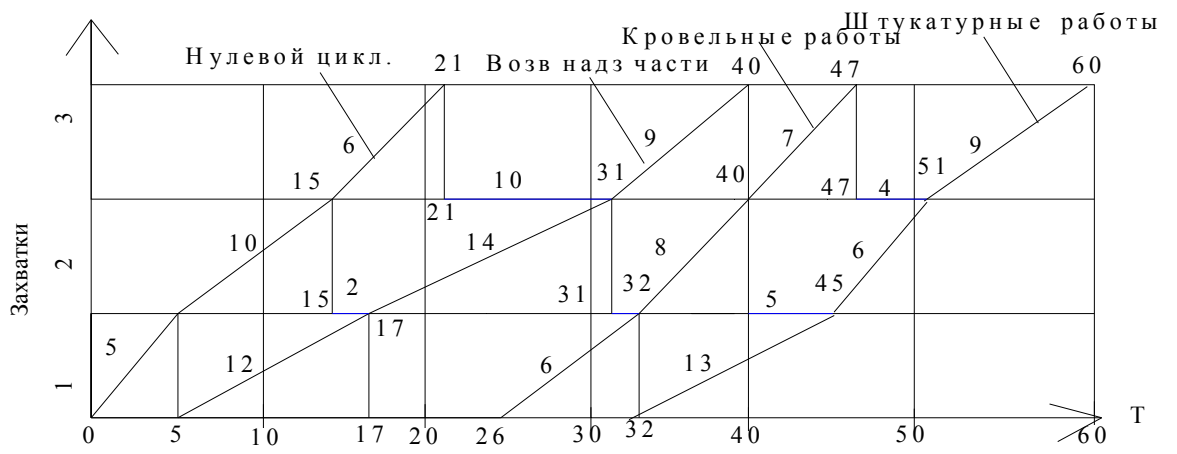
Рис. 5.1.(б) Циклограмма выполнения комплекса работ
