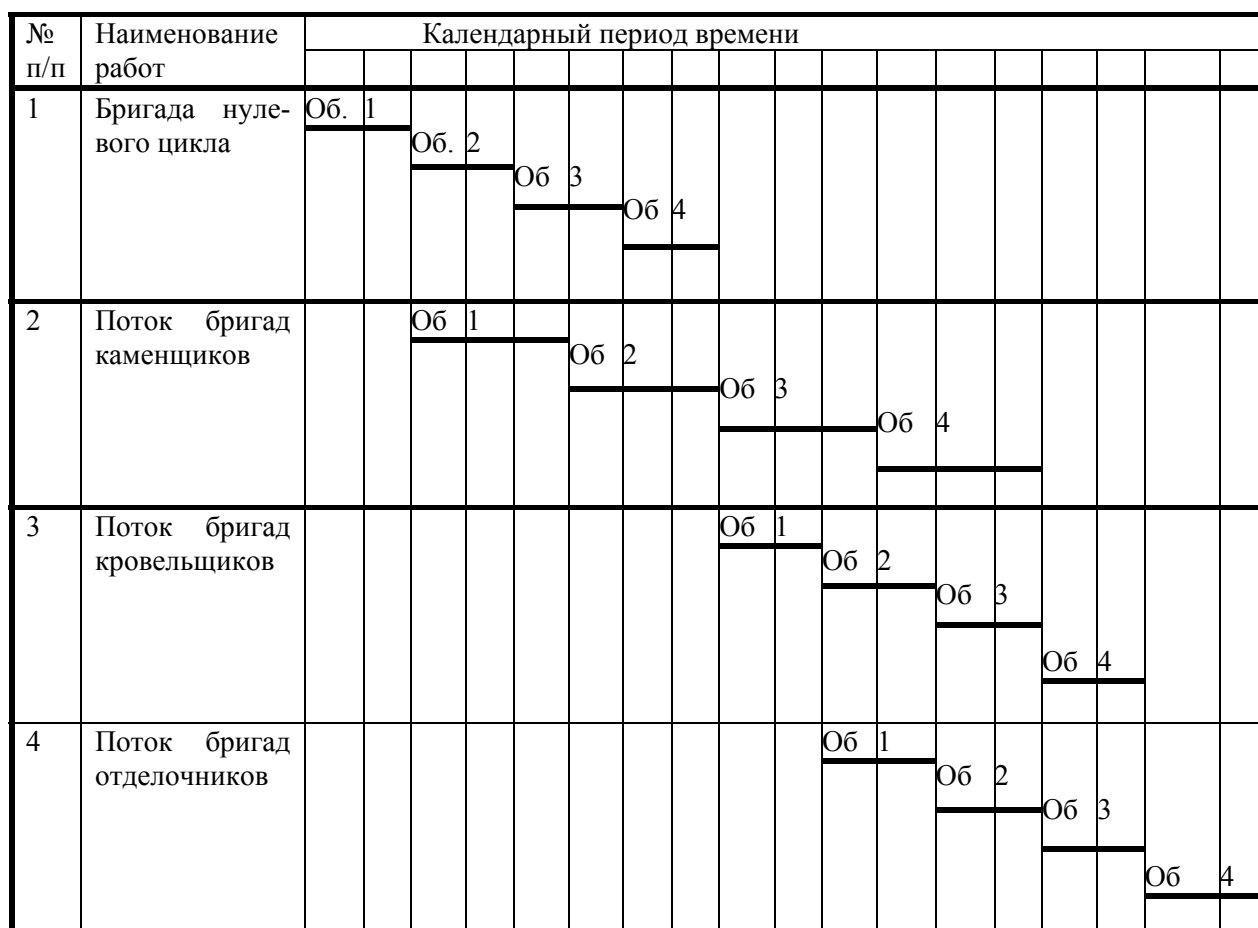
Рис. 3. Схема изображения поточного ведения работ в виде линейного графика
