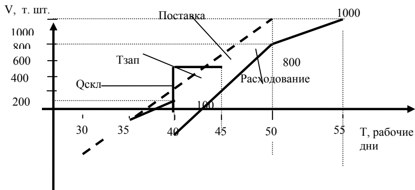
Рис. 4.4 Интегральный график при неравномерном расходе кирпича и равномерной поставке.
