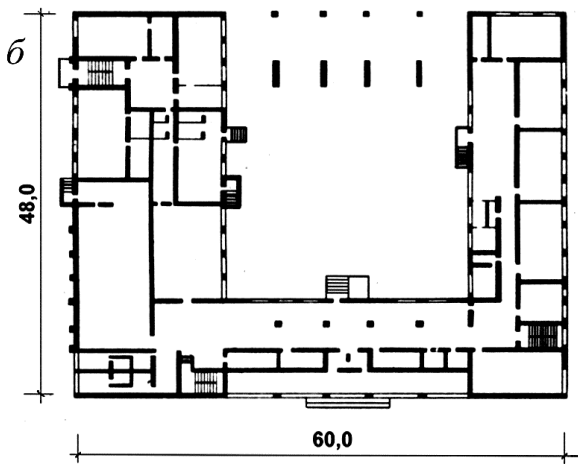
Рис. 24. Средняя общеобразовательная школа на 11 классов (320 учащихся): a – участок школы: 1 – школа; 2 – хозяйственный сарай; 3 – участок для цветочно-декоративных растений; 4 – метеорологическая и географическая площадка; 5 – участок для начальных классов; 6 – легкоатлетическая площадка; 7 – спортплощадки; 8 – гимнастическая площадка; 9 – мусоросборники; б – план первого этажа; в – план второго этажа
