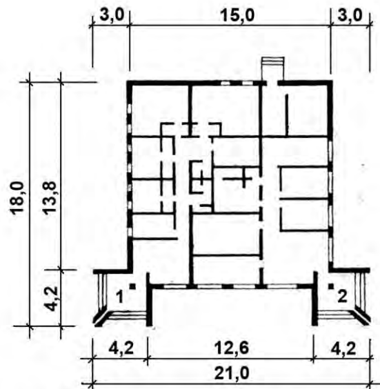
Рис. 27. Комбинат бытового обслуживания на 5 рабочих мест и гостиница на 6 мест: 1 – вход в гостиницу; 2 – вход в комбинат
