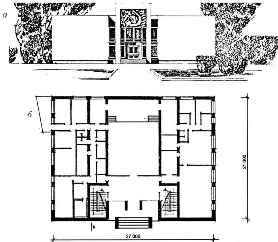
Рис. 10. Административное здание: a – фасад; б – план первого этажа
