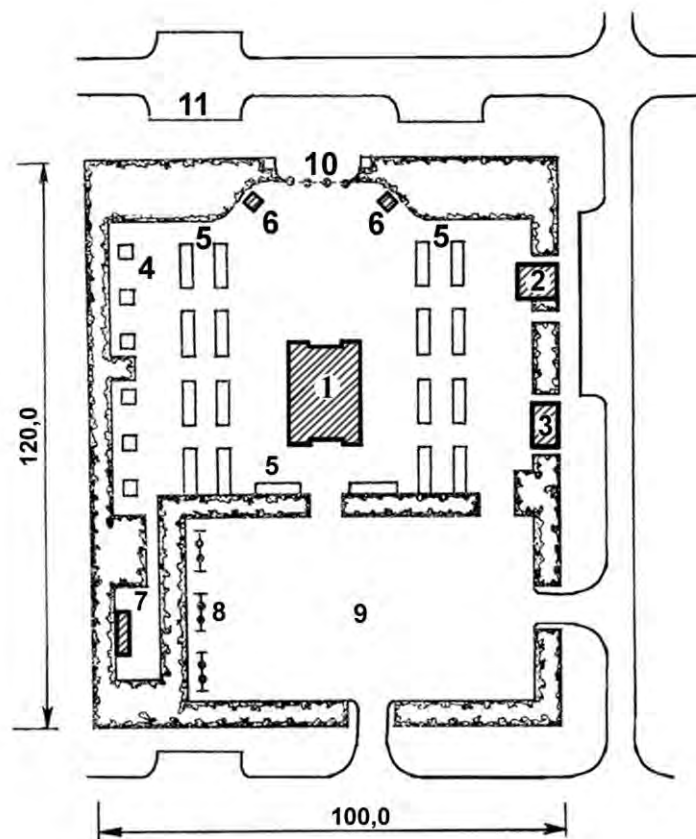
Рис. 28. Рыночная площадь: 1 – павильон для смешанной торговли; 2 – административный корпус; 3 – мясо-молочная контрольная станция; 4 – торговые ларьки; 5 – столы для торговли с рук; 6 – газетные и аптечные киоски; 7 – туалет; 8 – коновязи; 9 – место для торговли с возов и машин; 10 – вход на рынок; 11 – площадки для стоянки транспорта
