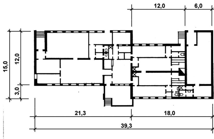
Рис. 31. Баня на 20 мест с прачечной самообслуживания на 200 кг сухого белья в смену
