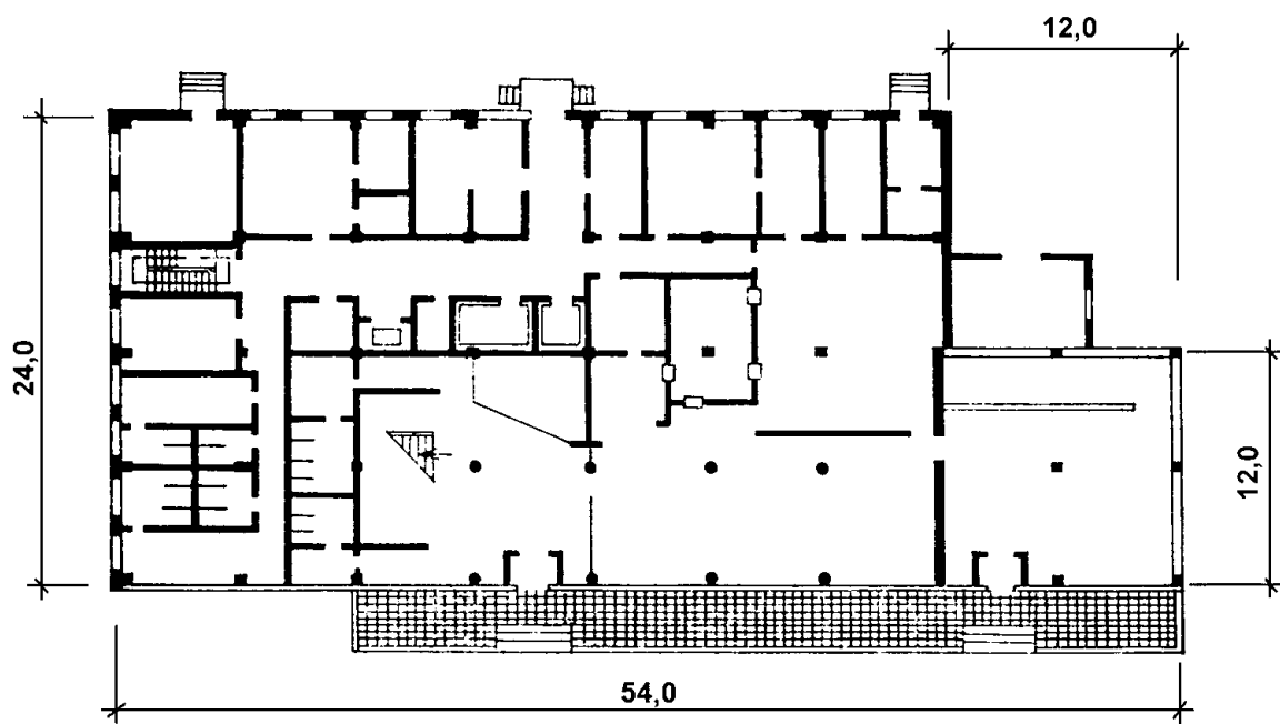
Рис. 15. Ресторан с кафе
