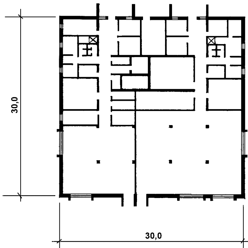
Рис. 14. Универмаг торговой площадью 400 м 2
