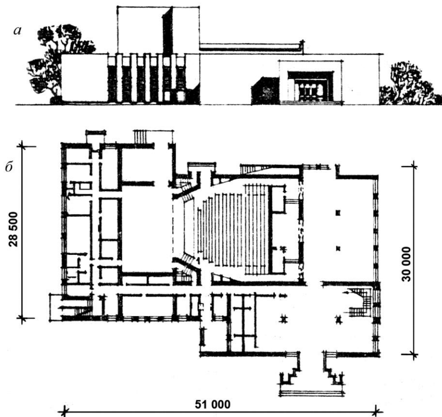
Рис. 11. Сельский дом культуры с залом на 500 мест: a – фасад; б – план первого этажа
