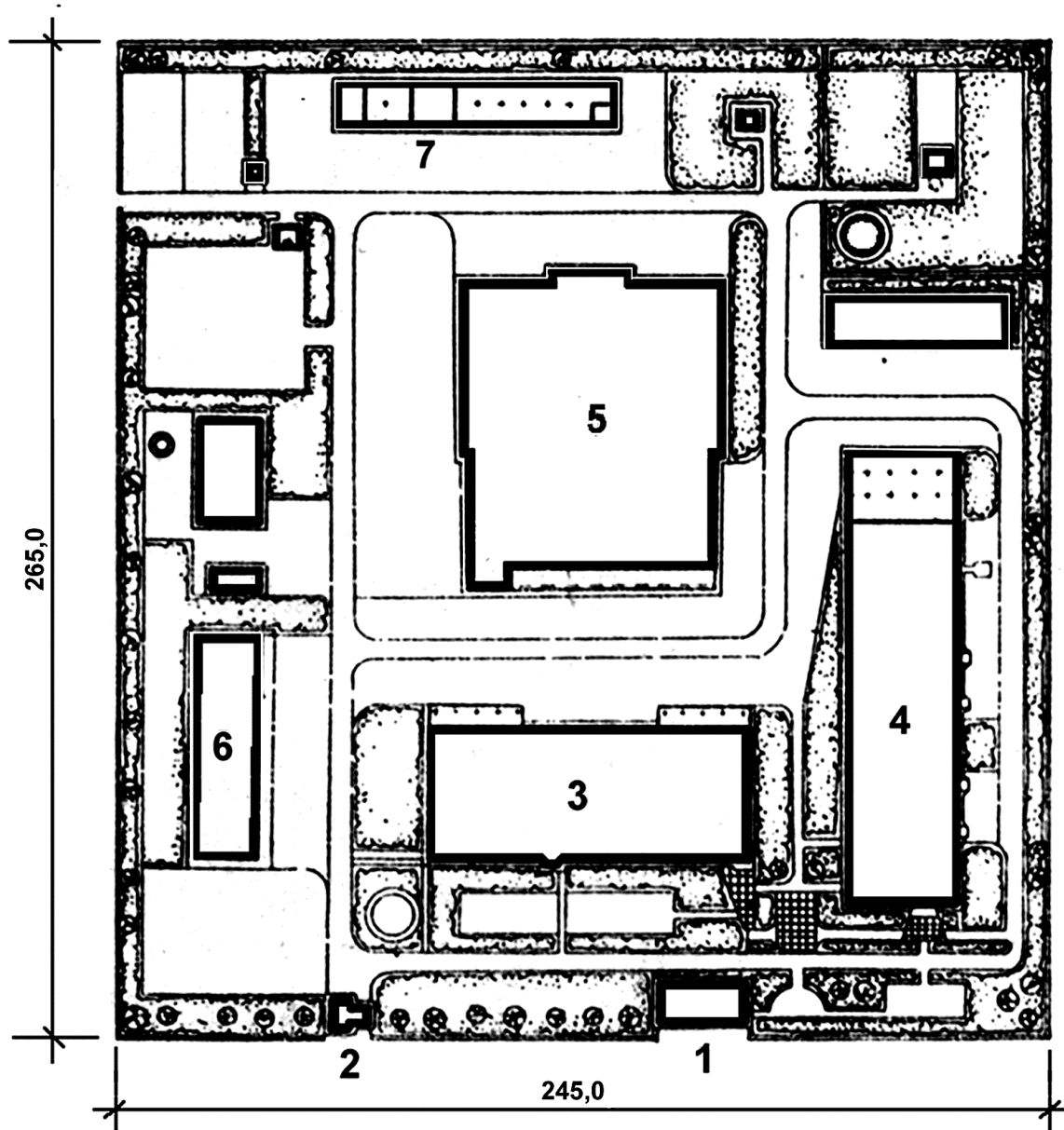
Рис. 34. Схема генерального плана плодокомбината: 1 – контора с проходной; 2 – проходная-весовая; 3 – цех плодово-ягодного виноделия; 4 – завод фруктовых консервов; 5 – фруктохранилище; 6 – склад готовой продукции; 7 – склад тары
