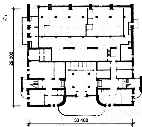
Рис. 25. Комплекс спортивных сооружений:
