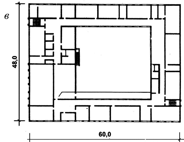
Рис. 24. Средняя общеобразовательная школа на 11 классов (320 учащихся): a – участок школы: 1 – школа; 2 – хозяйственный сарай; 3 – участок для цветочно-декоративных растений; 4 – метеорологическая и географическая площадка; 5 – участок для начальных классов; 6 – легкоатлетическая площадка; 7 – спортплощадки; 8 – гимнастическая площадка; 9 – мусоросборники; б – план первого этажа; в – план второго этажа
