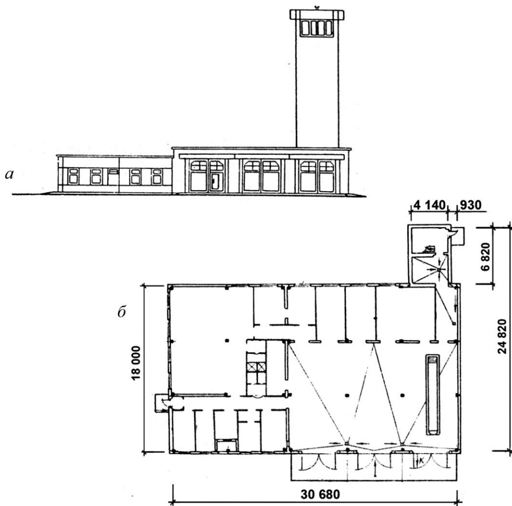
Рис. 32. Пожарное депо на 3 автомашины: а – фасад; б – план
