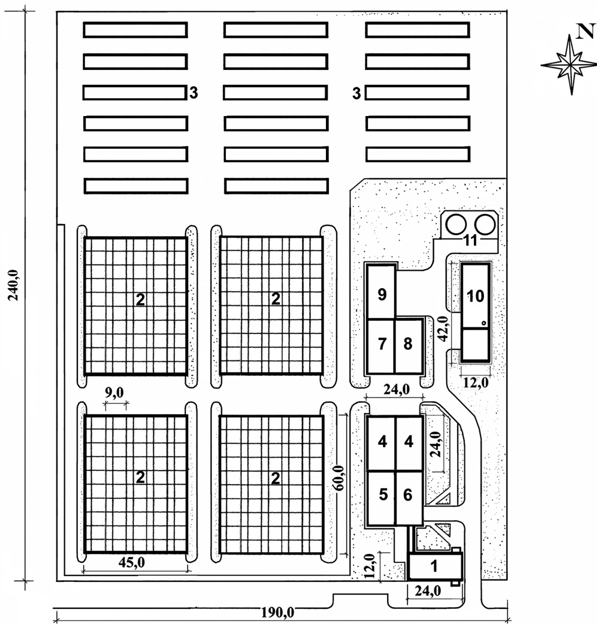
Рис. 33. План теплично-парникового комбината с котельной: 1 – административно-бытовой корпус с проходной; 2 – теплица; 3 – парники; 4 – склад продукции; 5 – цех по переработке; 6 – упаковочный цех; 7 – склад удобрений; 8 – склад оборудования и тары; 9 – гараж; 10 – котельная; 11 – склад ГСМ
