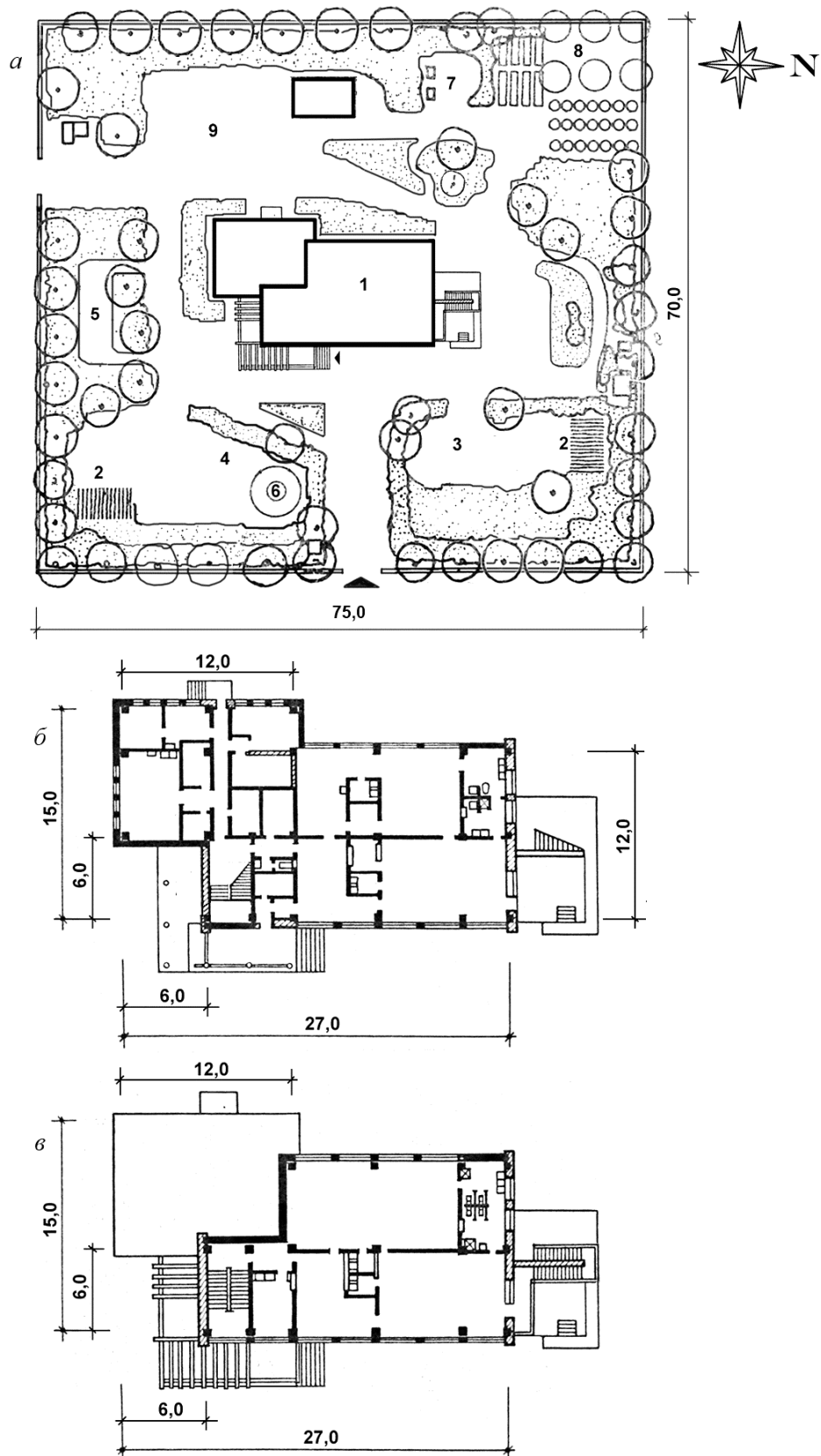
Рис. 26. Детское дошкольное учреждение на 45 мест (две группы): a – генплан участка: 1 – здание яслей-сада; 2 – теневой навес; 3 – групповая площадка ясельной группы; 4 – групповая площадка детского сада; 5 – физкультурная площадка; 6 – плескательный бассейн; 7 – площадка для животных и птиц; 8 – огород-ягодник; 9 – хозяйственный двор; б – план первого этажа; в – план второго этажа
