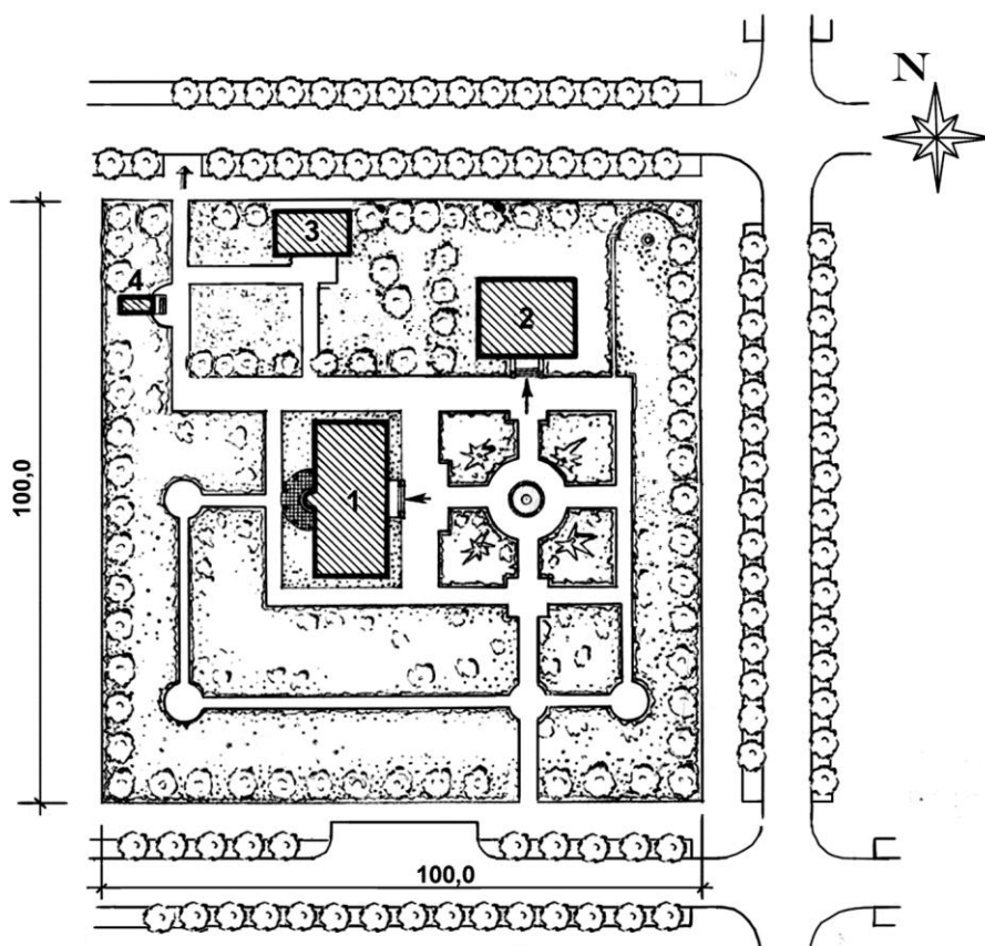
Рис. 29. Больница на 10 коек с врачебной амбулаторией: 1 – больница; 2 – амбулатория; 3 – хозяйственный корпус; 4 – морг
