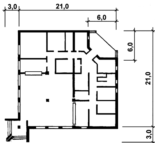
Рис. 13. Магазин товаров повседневного спроса
