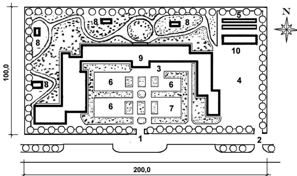
Рис. 30. Участок дома-интерната для престарелых: 1 – главный вход; 2 – хозяйственный въезд; 3 – вход в приемно-карантинное отделение; 4 – хозяйственная зона; 5 – парники; 6 – физкультурные площадки; 7 – танцевально-игровая площадка; 8 – беседки, павильоны; 9 – главный корпус; 10 – хозяйственные сооружения
