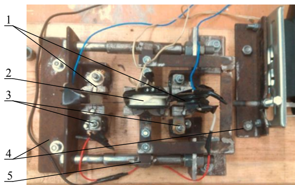
Рис. 4. Внешний вид макетного образца возвратно-поступательного электрического генератора
