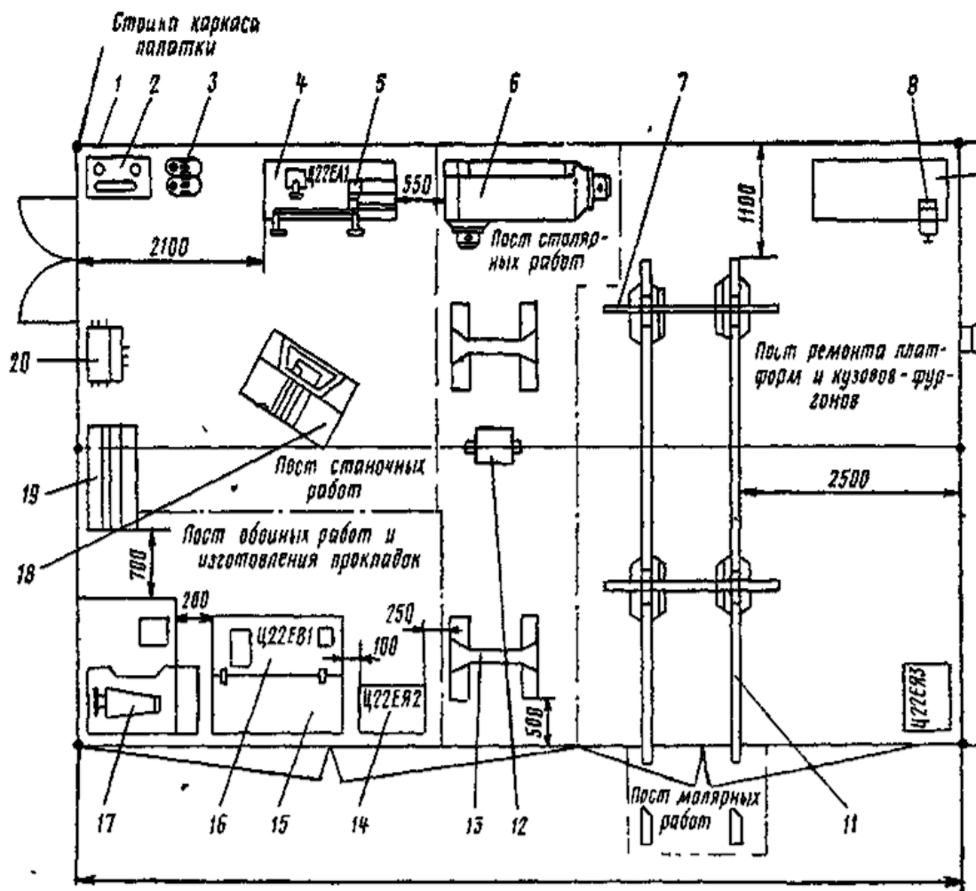
Рисунок 5.10 – Размещение оборудования отделения деревообделочных, обоевых и малярных работ Ц22Е:
