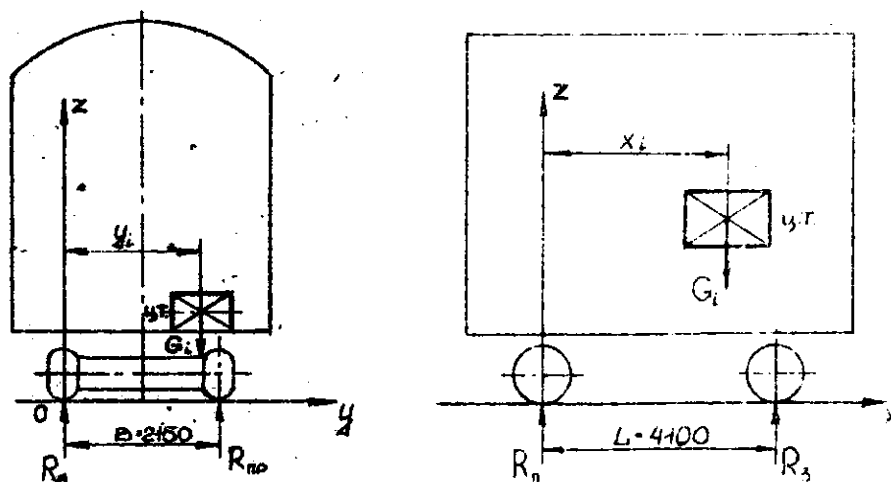
Рисунок 7.1 – Принципиальная схема распределения нагрузок
