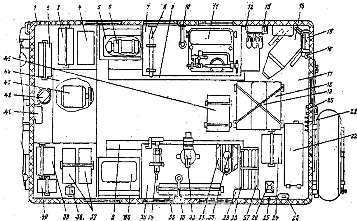
Рисунок 5.3 – Размещение оборудования и имущества в кузове мастерской MPC-AT-M1:
