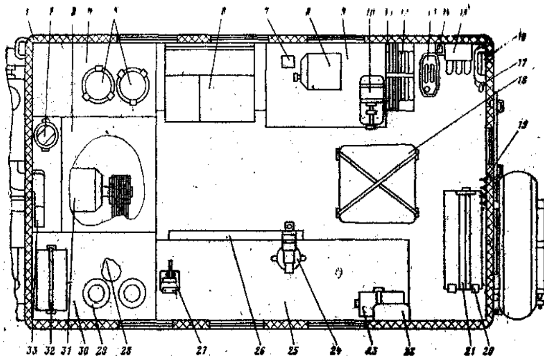
Рисунок 5.8 – Размещение оборудования и имущества в кузове ремонтно-зарядной аккумуляторной станции СРЗ-А-М1:
