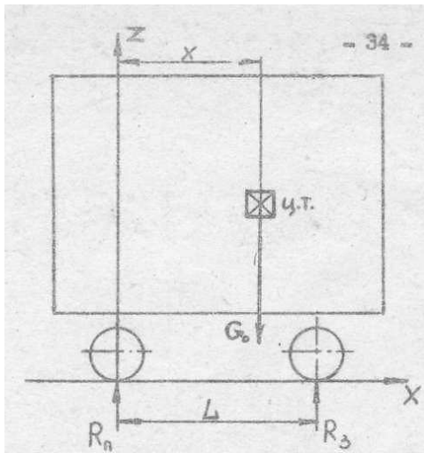
Рисунок 7.2 – Схема распределения сил для определения координат центра тяжести
