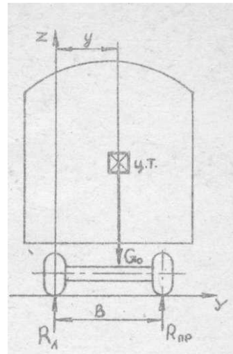
Рисунок 7.2 – Схема распределения сил для определения координат центра тяжести
