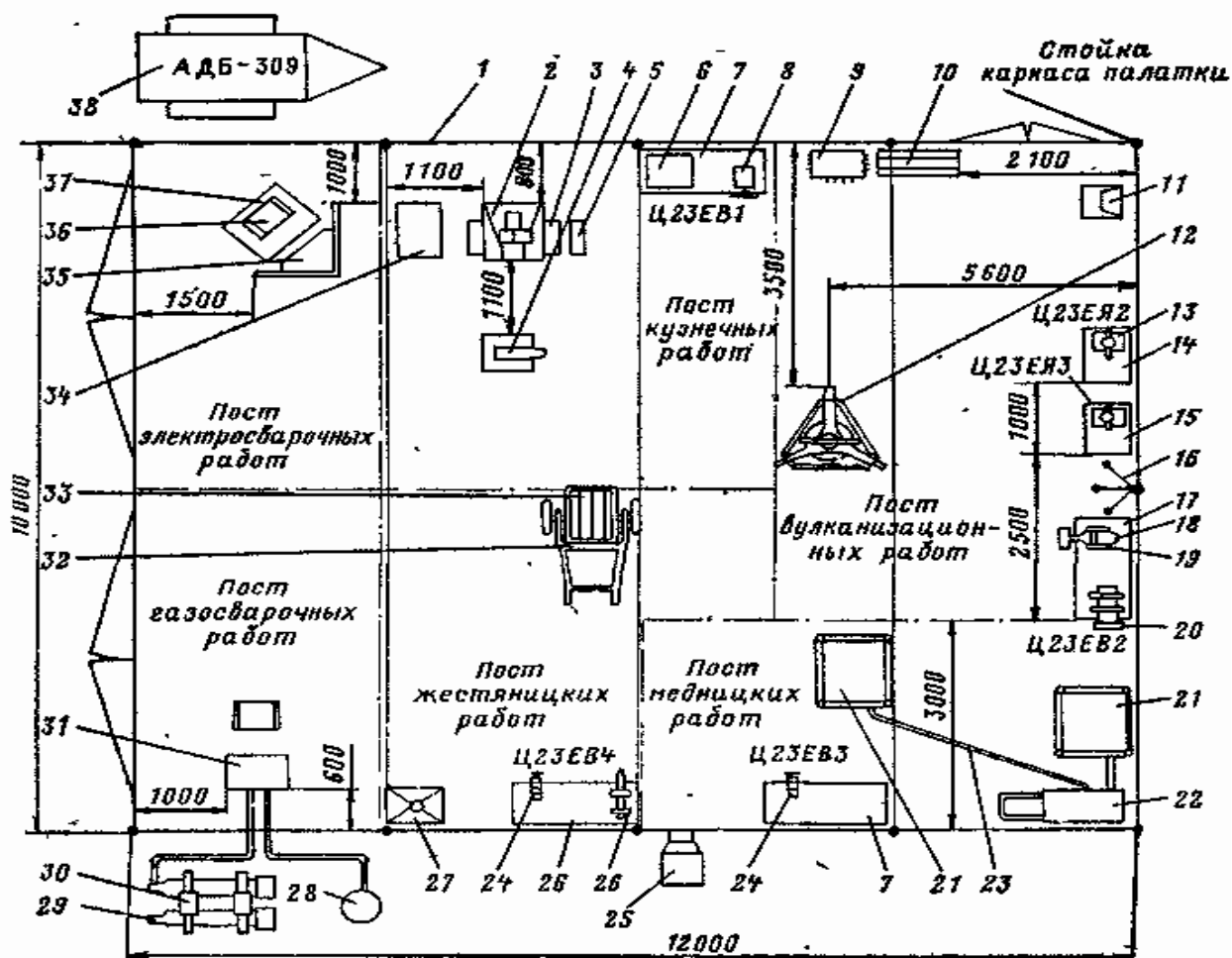
Рисунок 5.11 – Размещение оборудования отделения тепловых работ Ц23Е:
