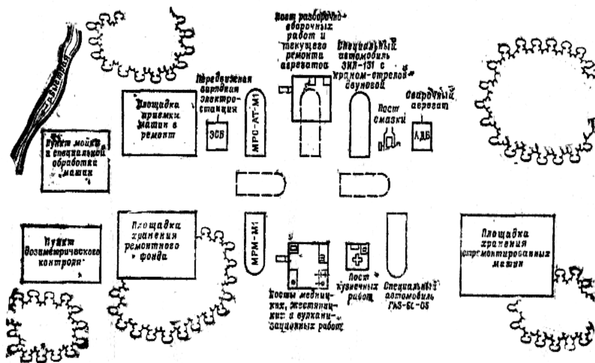
Рисунок 2.3 – Схема размещения на местности материальной части ПАРМ-1М1-4ОС
