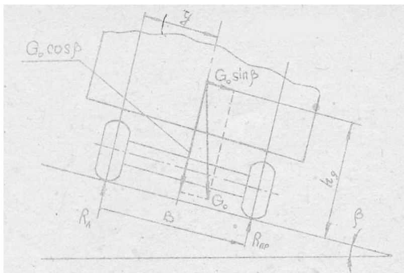
Рисунок 7.5 – Схема распределения сил при расчете мастерской на боковое опрокидывание
