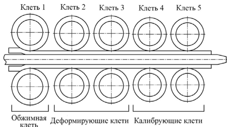
Рис. 2. Схема расположения клетей непрерывного раскатного стана
