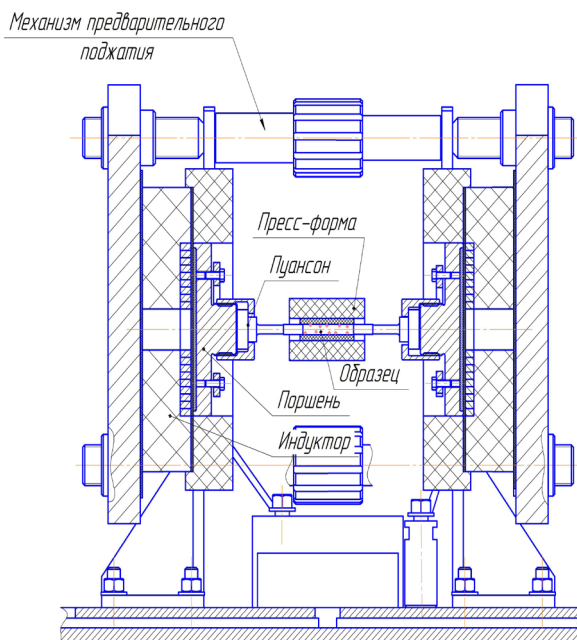
Рис. 2. Конструкция блока технологического
