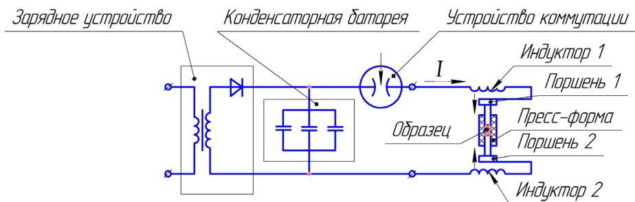
Рис. 1. Электрическая схема процесса комбинированного прессования и спекания
