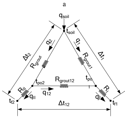
Рис. 3. Эквивалентные схемы процесса: а –используемая; б – по [1]
