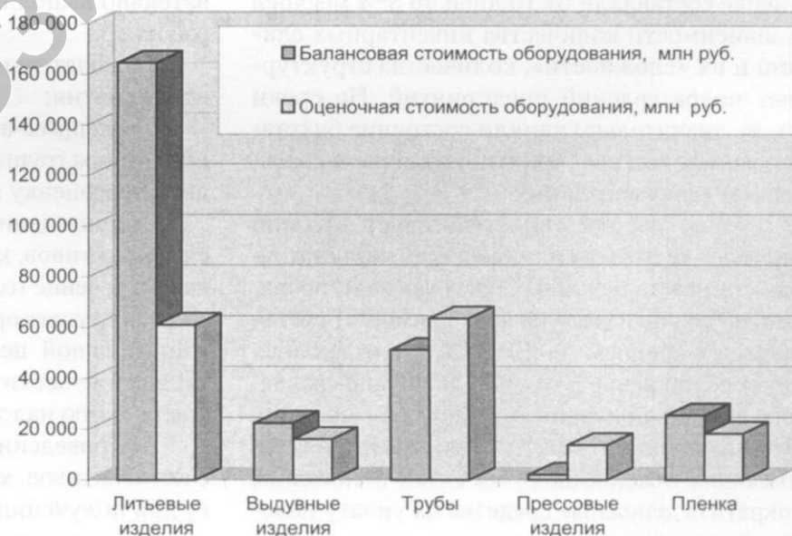
Рис. 1. Соотношение результатов прямой и индексной оценки оборудования по производству различных изделий.
