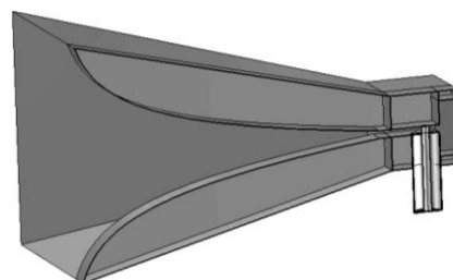
Рис. 10. Конструкция рупора на основе Н-образного волновода (в разрезе)
