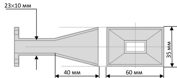
Рис. 1. Пирамидальный рупорный облучатель
