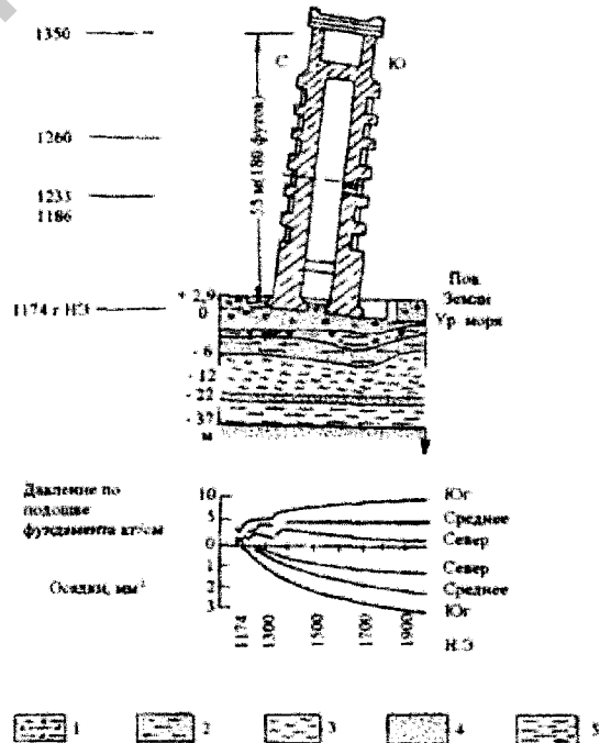
Рис. 3. Пизанская башня: 1 – серые глинистые алевролиты; 2 – глинистые пески; 3 – голубые глины; 4 – пески; 5 – известняк
