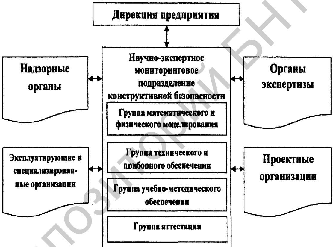
Рис. 8. Организационно-техническая схема системы технического мониторинга объекта
