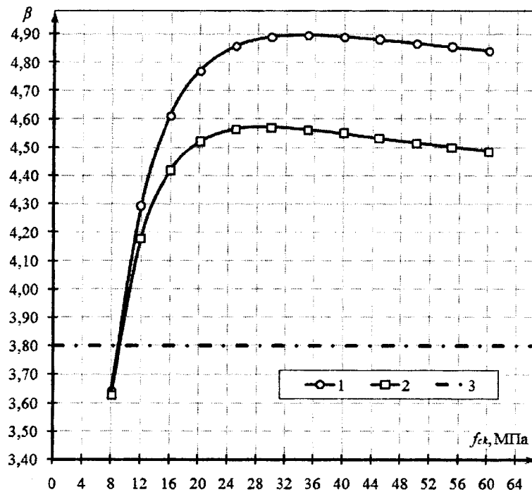
Рис. 5. Зависимость значений индекса надежности \beta от значений прочности бетона f_{ck} : 1 – расчет по [1]; 2 – расчет по [2]; 3 – линия \beta = 3,8
