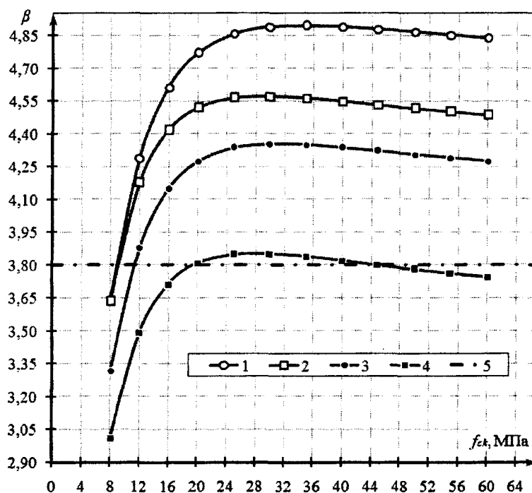
Рис. 6. Зависимость значений индекса надежности \beta от значений прочности бетона f_{ck} : 1 – расчет по [1] при C_{Rd,c} = 0,225 ; 2 – расчет по [2]; 3 – расчет по [1] при C_{Rd,c} = 0,24 ; 4 – расчет по [1] при C_{Rd,c} = 0,255 ; 5 – линия \beta = 3,8
