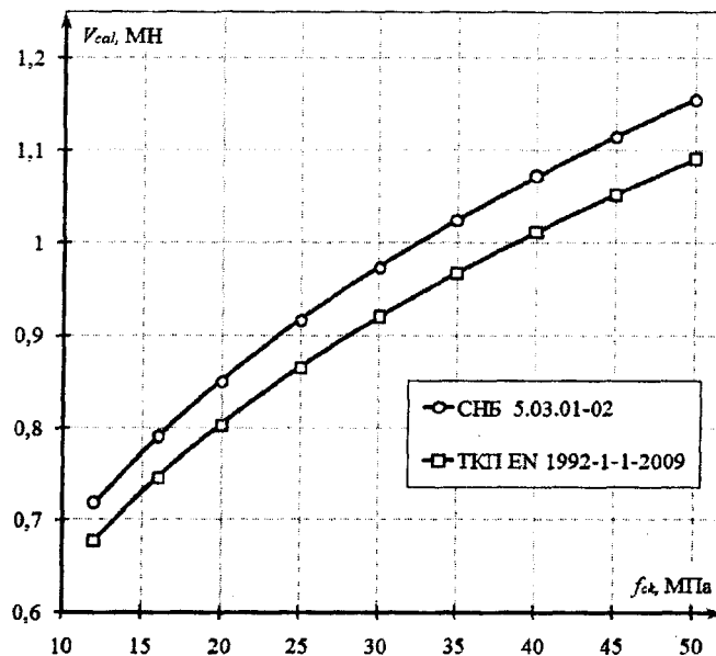
Рис. 1. Изменение значений разрушающих усилий при местном срезе V_{cal} в зависимости от прочности бетона f_{ck} (при d = 200 мм и \rho = 0,01 ) для норм [1, 2]
