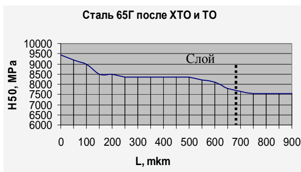
Рисунок 1 – Распределение микротвердости на стали 65Г.
